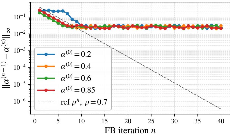
FB-PDE convergence (N=100, milan)
