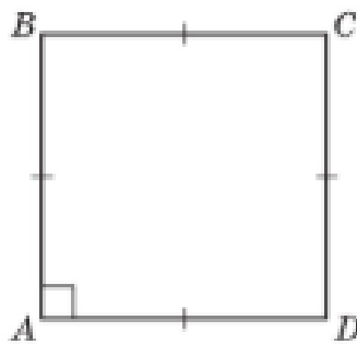
Рис. 1. Квадрат ABCD
