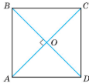
Рис. 2. Діагоналі квадрата
