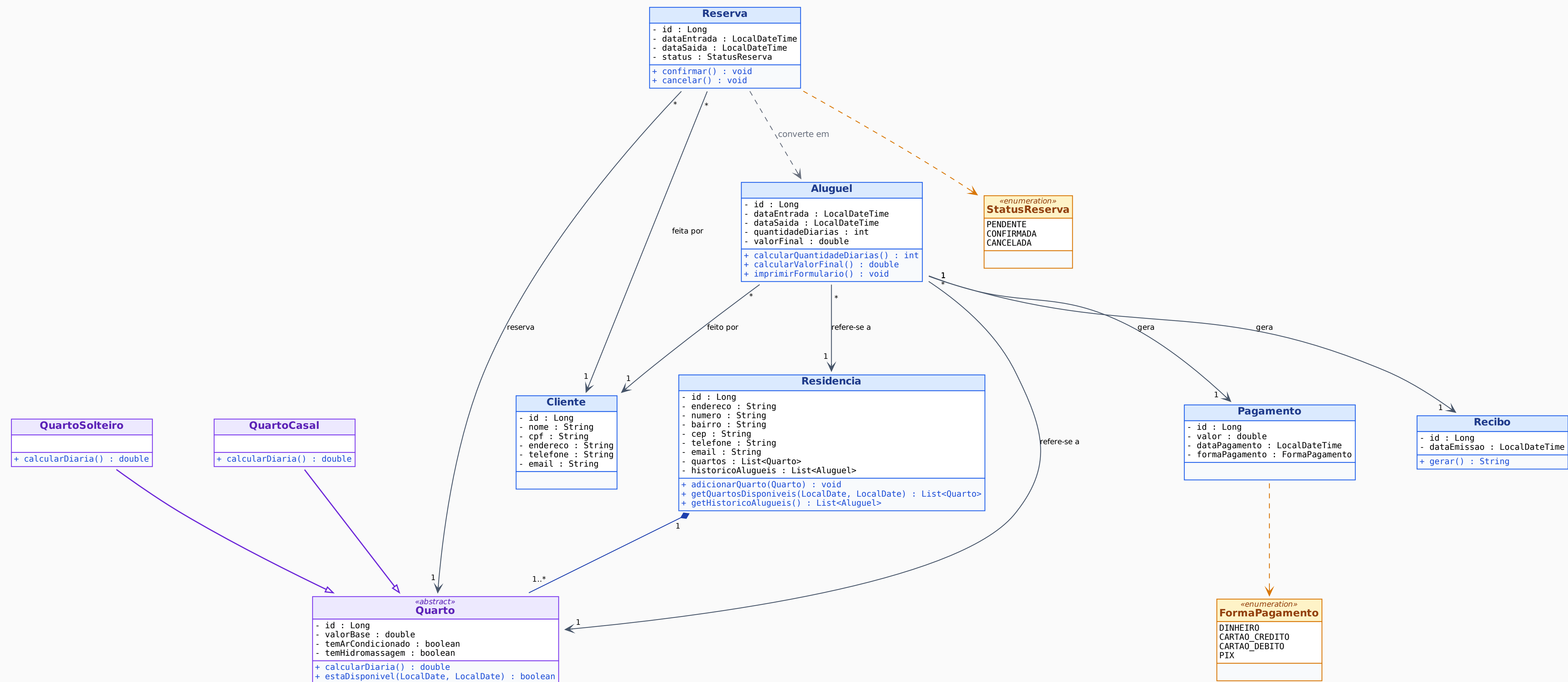
Sistema de Hospedagem — Diagrama de Classes
