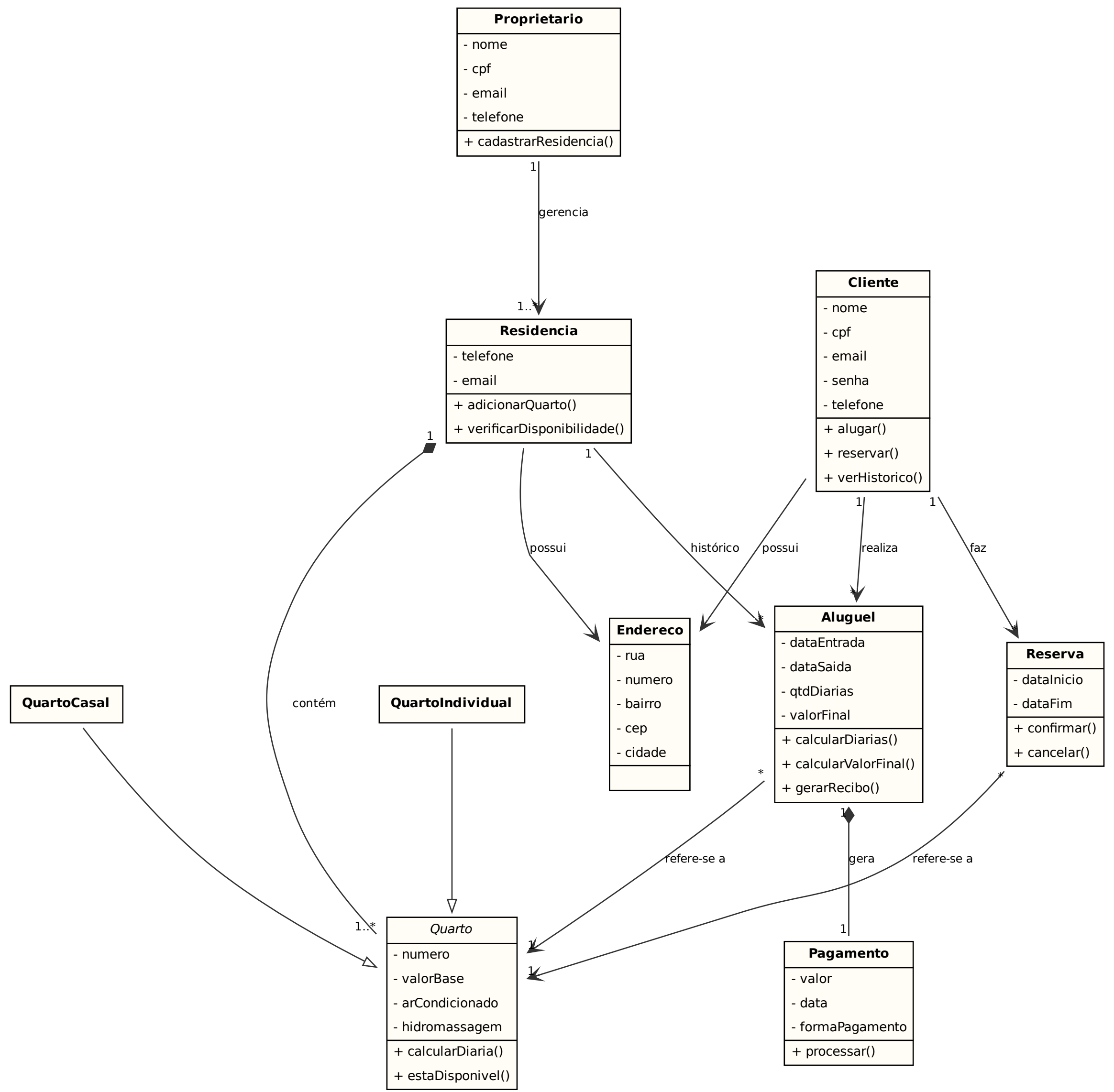
Diagrama de Classes — Sistema de Hospedagem Maraú
