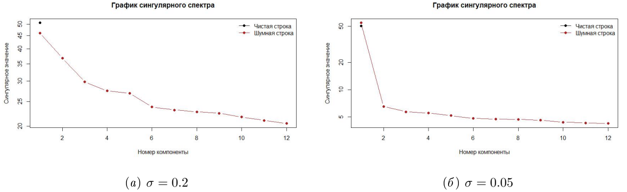
Рис. 2.2. Первые двенадцать сингулярных значений для чистой и зашумленной строки длины n = 100 после дискретного преобразования Фурье
