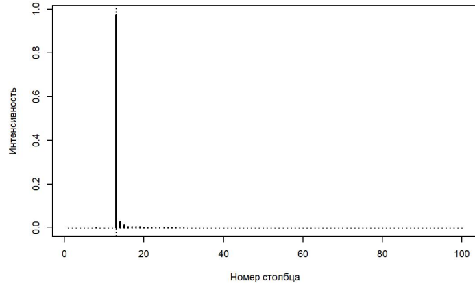
Та же строка при \sigma = 0.05 , строка 39
