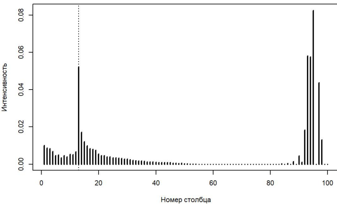
Растекание около верного пикселя, строка 39
