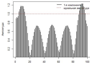
Амплитуда компоненты
