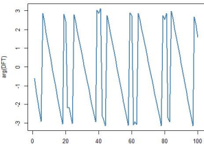
Фаза компоненты
