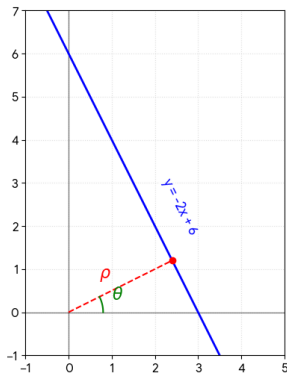
Рис. 2. Параметризация прямой через \rho и \theta
