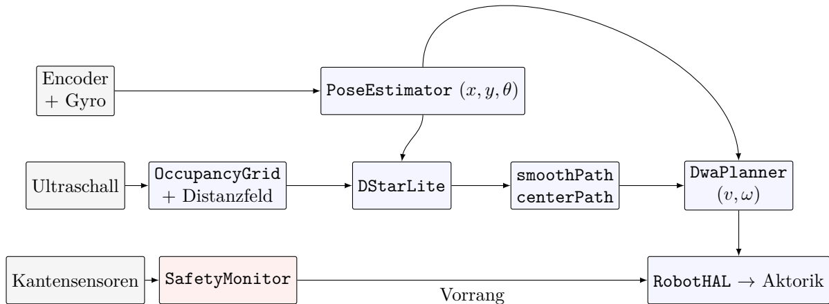
Abbildung 2: Datenfluss in MODE_SIM_TEST . Die Sicherheitskomponente wird in jedem Regelzyklus vor der Navigation ausgewertet und übernimmt bei einem Kantenereignis die Aktorik.
