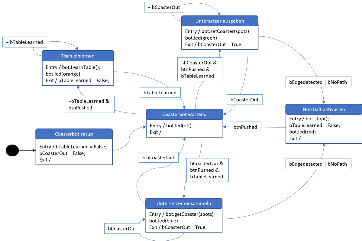
Abbildung 3: Ablauf für die Missionsablaufsteuerung des Coasterbot-Prototyps: sechs Zustände ( Coasterbot setup , Coasterbot wartend , Tisch einlernen , Untersetzer ausgeben , Untersetzer einsammeln , Not-Halt aktivieren ) mit Entry-/Exit-Aktionen (LED-Farbe, bot.LearnTable() , bot.setCoaster() , bot.getCoaster() , bot.stop() ) und Wächterbedingungen auf den Flags bTableLearned , bCoasterOut , btnPushed sowie den Fehlersignalen bEdgedetected / bNoPath .
