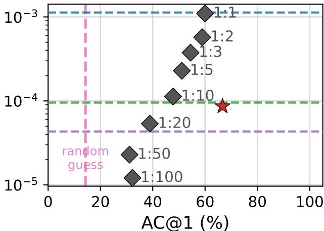
RE2-OB — TraceRCA (AC@1)
