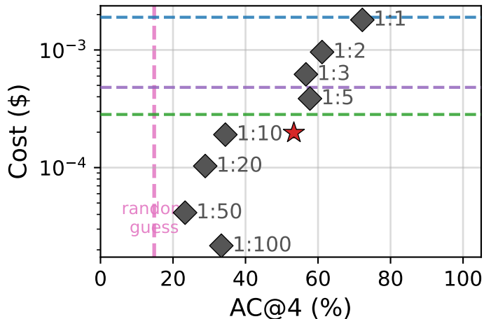
RE2-TT — TraceRCA (AC@4)
