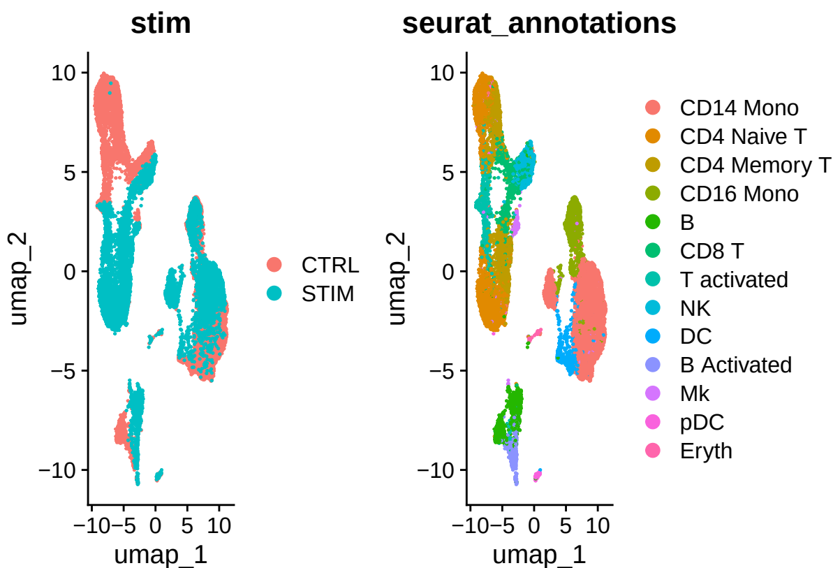
Figure 5: UMAP-visualisatie na SCTransform-normalisatie. Cellen zijn gekleurd op basis van conditie en celtype. De figuur laat zien dat SCTransform een alternatieve methode biedt om technische variatie te corrigeren.
