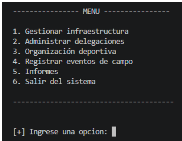
Imagen 2: Menú principal
