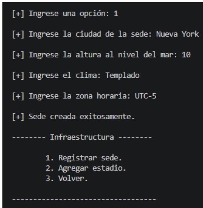
Imagen 3.1: Registrar sede
