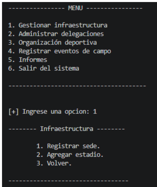
Imagen 3: Gestionar infraestructura
