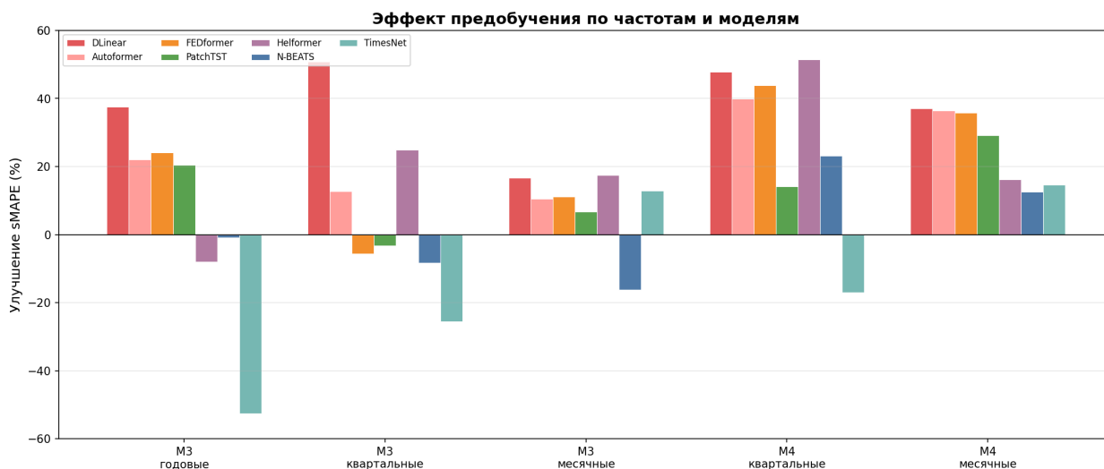
Рисунок 17. Эффект предобучения: относительное улучшение sMAPE (%) по частотам и моделям
