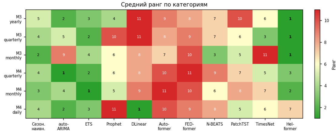
Рисунок 14. Тепловая карта рангов: модели × категории
