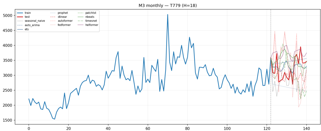
Рисунок 8. Пример прогноза на месячном ряде T779 набора M3
