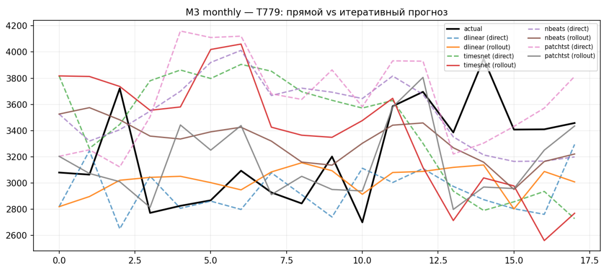
Рисунок 16. Сравнение прямого и итеративного прогнозов на месячном ряде T779
