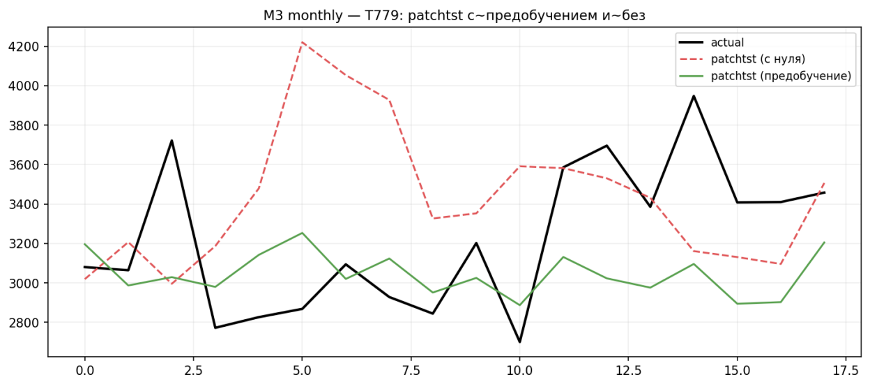
Рисунок 18. PatchTST: прогноз с предобучением и без на ряде T779
