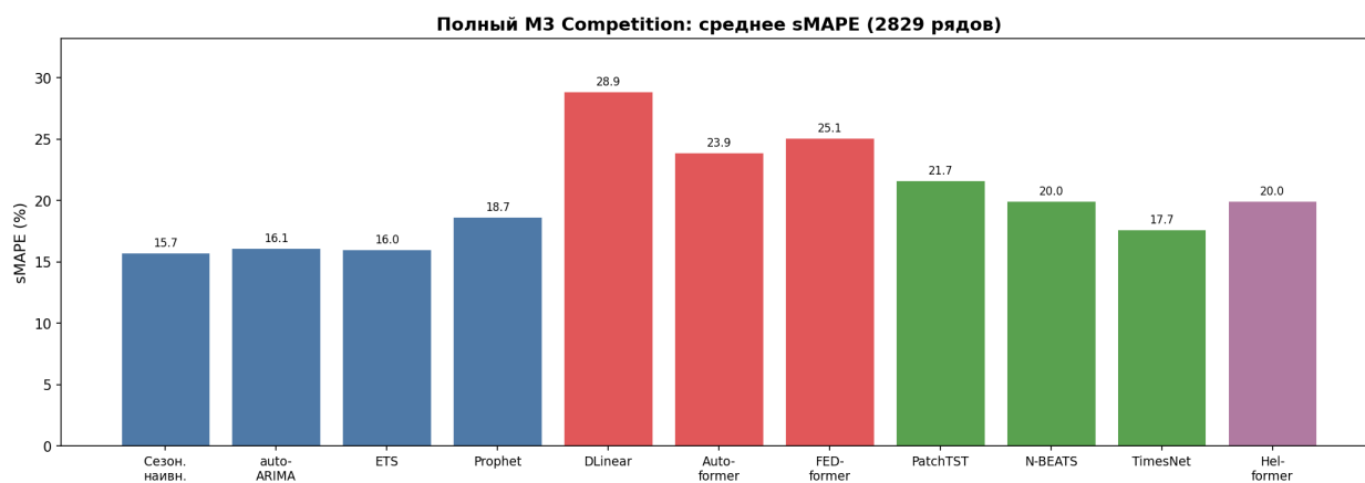
Рисунок 5. Среднее sMAPE на полном M3 Competition (2829 рядов, 11 моделей)
