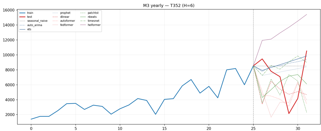
Рисунок 6. Пример прогноза на годовом ряде T352 набора M3
