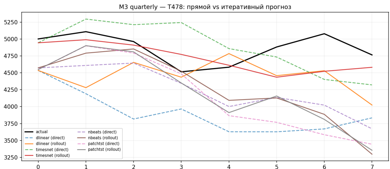
Рисунок 15. Сравнение прямого и итеративного прогнозов на квартальном ряде T478
