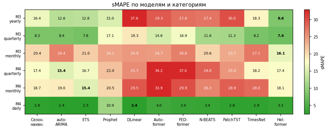
Рисунок 13. Тепловая карта sMAPE: модели × категории
