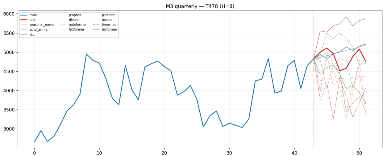
Рисунок 7. Пример прогноза на квартальном ряде T478 набора M3
