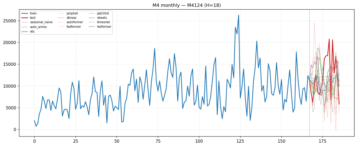
Рисунок 11. Предсказания 11 моделей на месячном ряде M4124 набора M4 Competition (горизонт H=18 )
