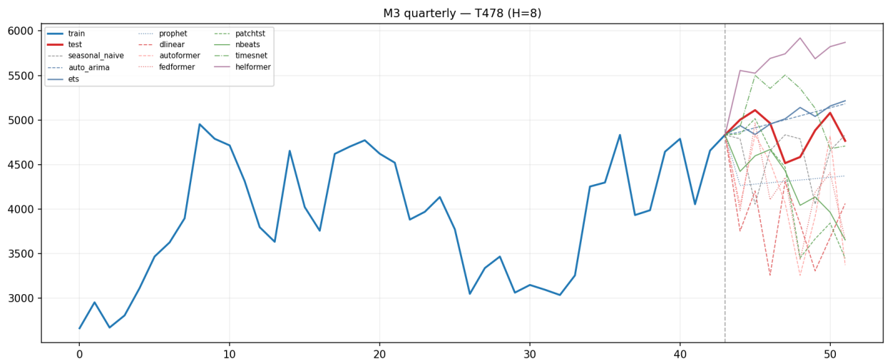
Рисунок 7. Предсказания 11 моделей на квартальном ряде T478 набора M3 Competition (горизонт H=8 )
