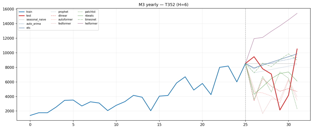
Рисунок 6. Предсказания 11 моделей на годовом ряде T352 набора M3 Competition (горизонт H=6 )
