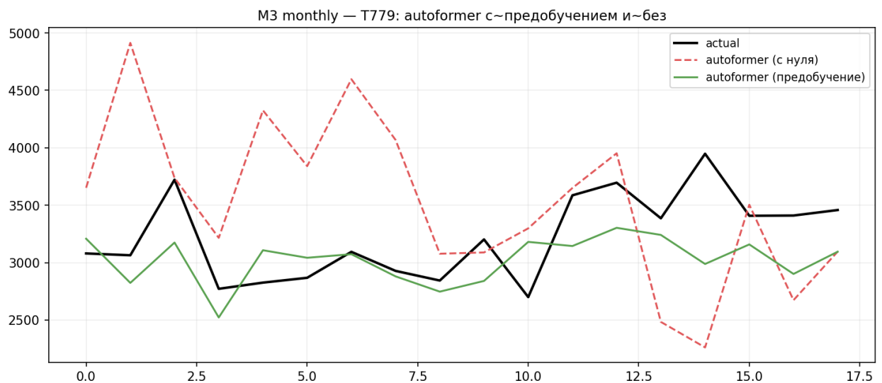
Рисунок 19. Предсказания Autoformer с предобучением и без на месячном ряде T779 набора M3 Competition (горизонт H=18 )
