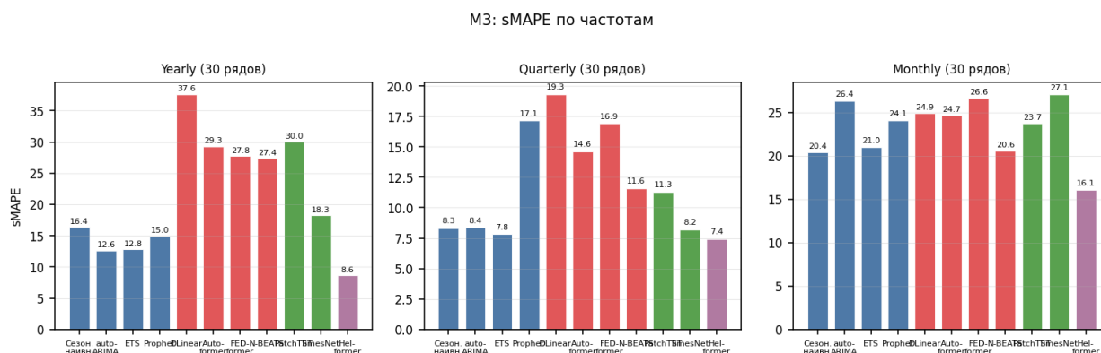
Рисунок 4. Распределение sMAPE (%) по частотным категориям M3 Competition для 11 моделей (подвыборка 30 рядов на категорию)
