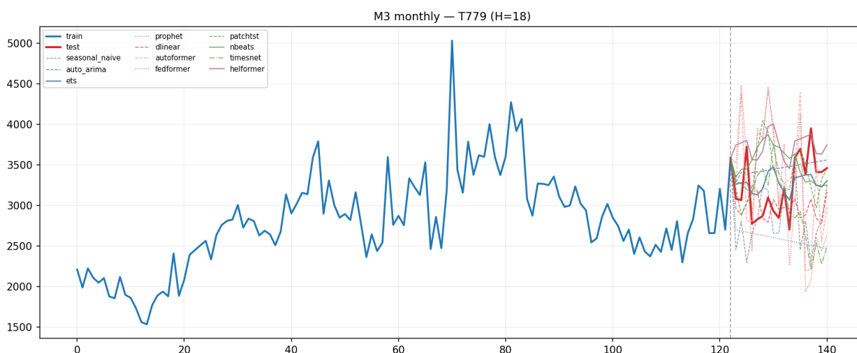
Рисунок 8. Предсказания 11 моделей на месячном ряде T779 набора M3 Competition (горизонт H=18 )
