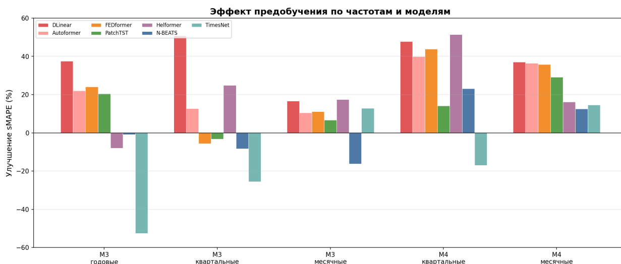
Рисунок 17. Эффект предобучения: относительное улучшение sMAPE (%) для 7 нейросетевых моделей по пяти частотным категориям M3 и M4 Competition
