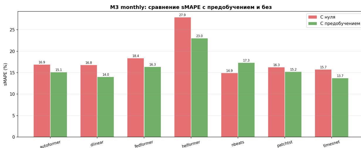
Рисунок 18. Сравнение sMAPE моделей с предобучением и без на месячных рядах M3 Competition
