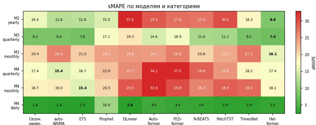
Рисунок 12. Тепловая карта sMAPE (%) для 11 моделей по шести частотным категориям M3 и M4 Competition
