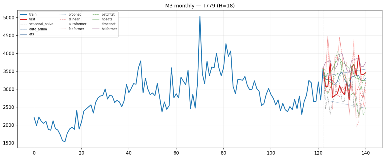
Рисунок 7. Предсказания 11 моделей на месячном ряде T779 набора M3 Competition (горизонт H=18 )
