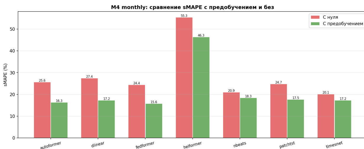
Рисунок 20. Сравнение sMAPE моделей с предобучением и без на месячных рядах M4 Competition
