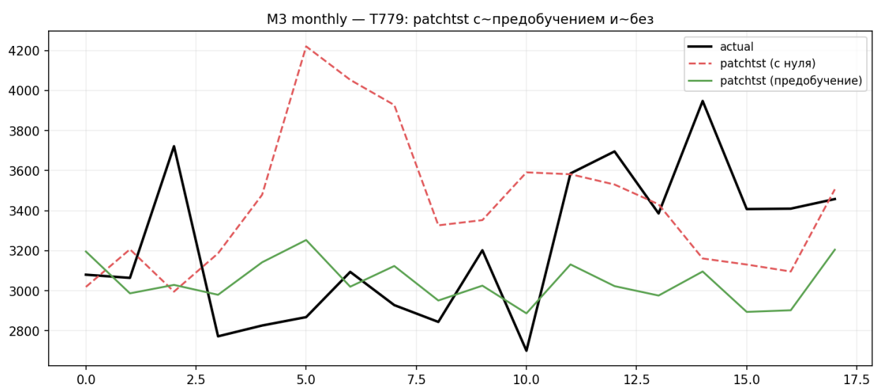
Рисунок 22. Предсказания PatchTST с предобучением и без на месячном ряде T779 набора M3 Competition (горизонт H=18 )
