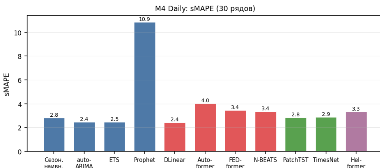
Рисунок 8. Распределение sMAPE (%) на ежедневных рядах M4 Competition для 11 моделей (30 рядов, горизонт H=14 )
