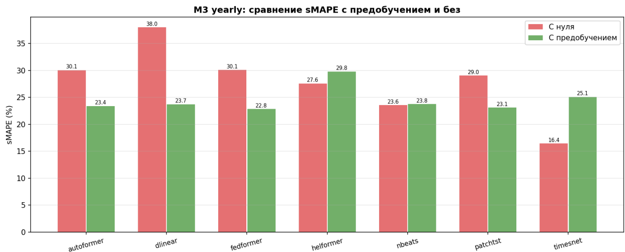
Рисунок 16. Сравнение sMAPE моделей с предобучением и без на годовых рядах M3 Competition
