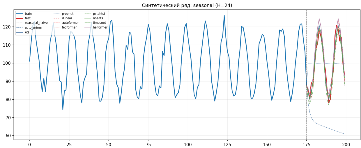
Рисунок 1. Предсказания 11 моделей на синтетическом ряде с чистой сезонностью (200 наблюдений, H=24 )
