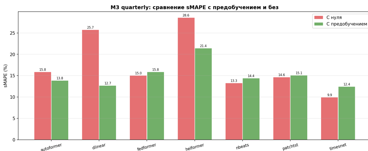
Рисунок 17. Сравнение sMAPE моделей с предобучением и без на квартальных рядах M3 Competition
