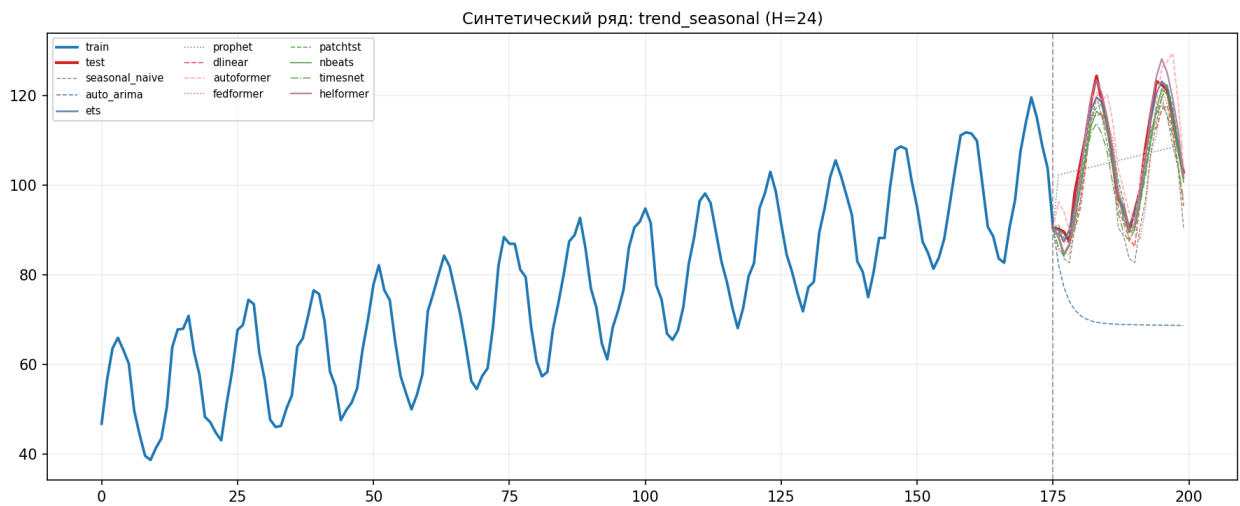
Рисунок 2. Предсказания 11 моделей на синтетическом ряде с трендом и сезонностью (200 наблюдений, H=24 )
