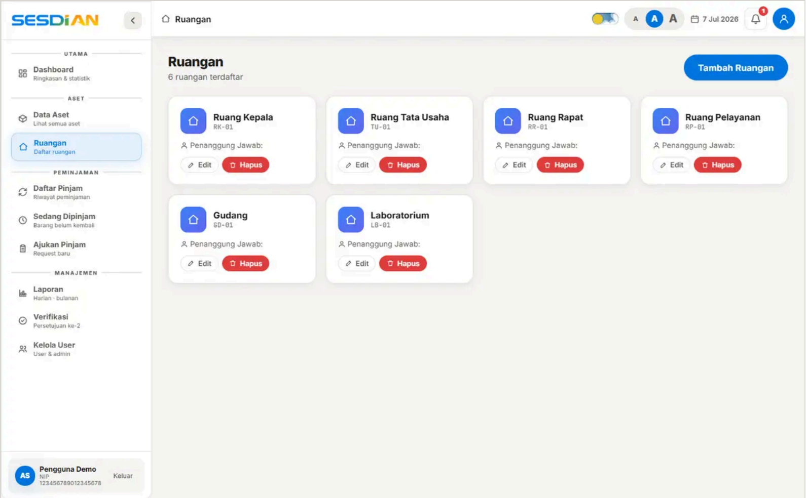
Gambar F.4. Halaman Kelola Ruangan
