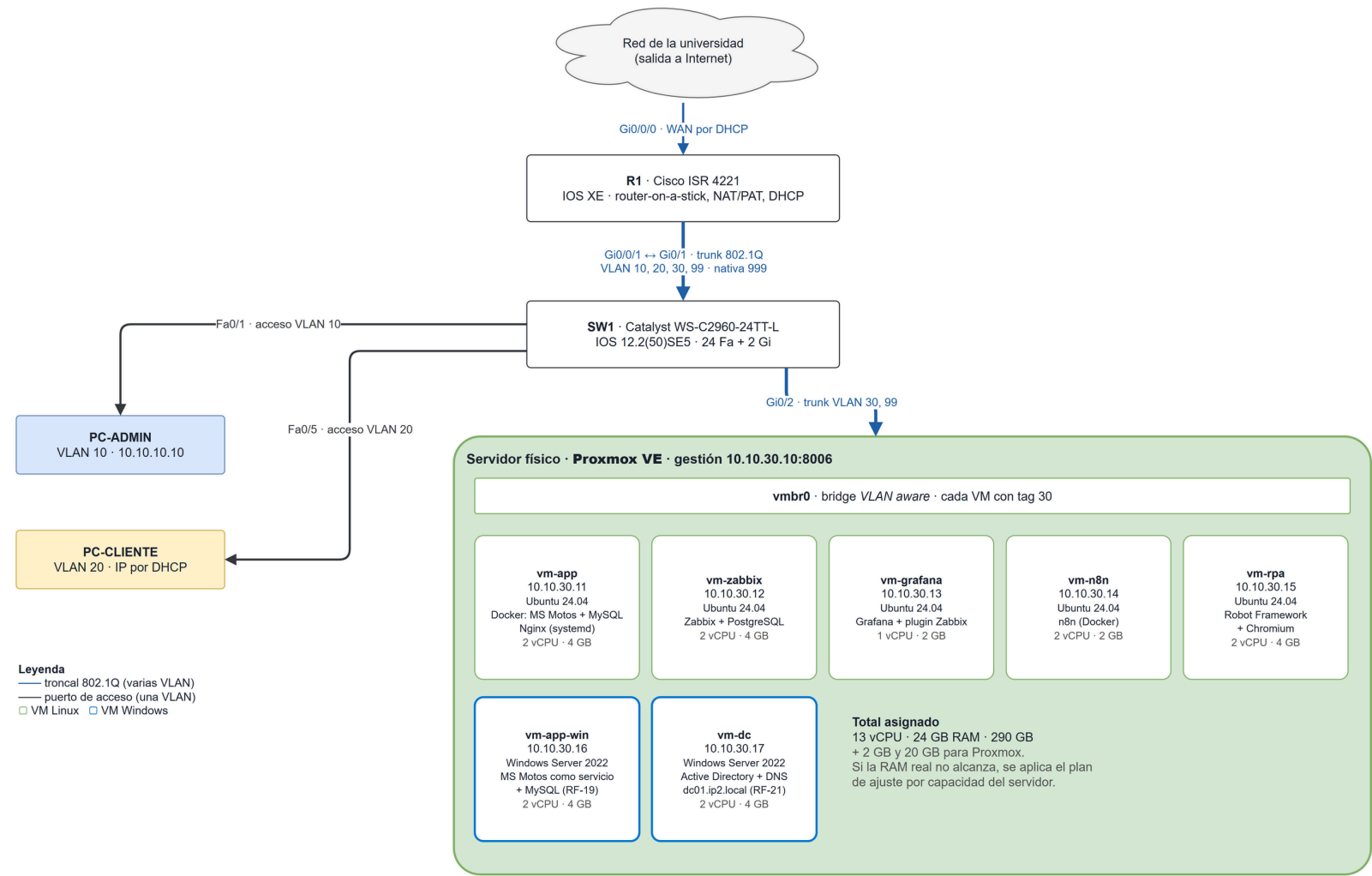
Figura 1 · Arquitectura física: qué se cablea con qué. Fuente editable: docs/diagramas/arquitectura-fisica.drawio
