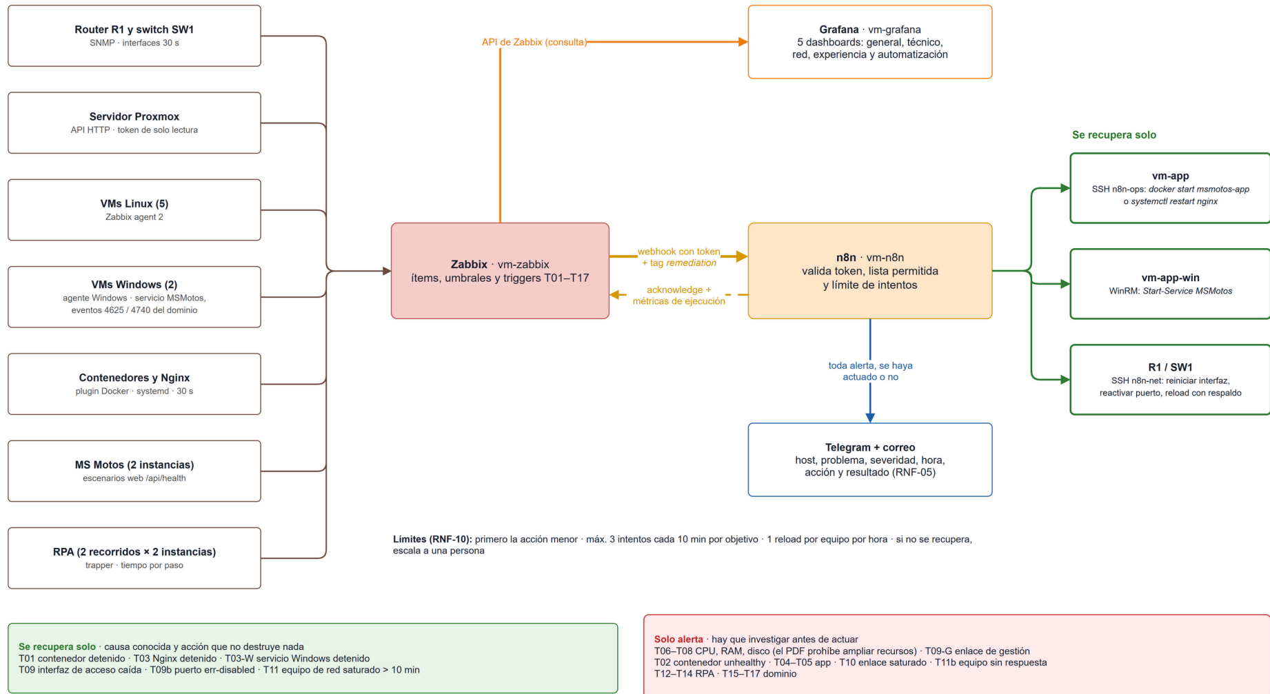
Figura 4 · Monitoreo y automatización: qué vigila Zabbix, qué recupera n8n y qué solo alerta. Fuente editable: docs/diagramas/flujo-monitoreo.drawio
