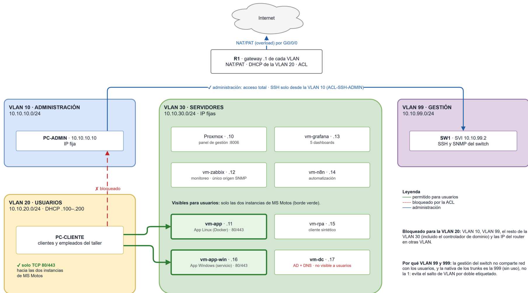
Figura 2 · Arquitectura lógica: segmentación y tráfico permitido. Fuente editable: docs/diagramas/arquitectura-logica.drawio
