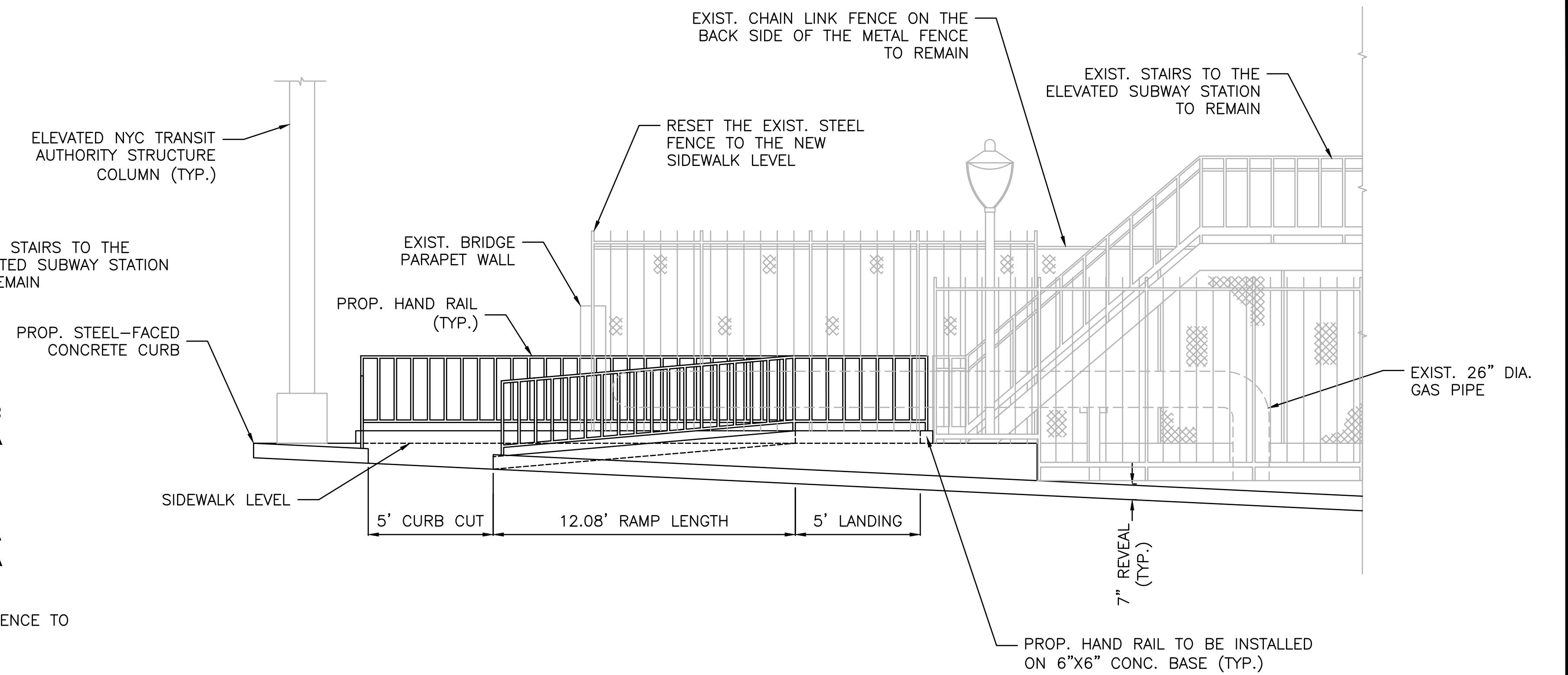
SECTION A-A
