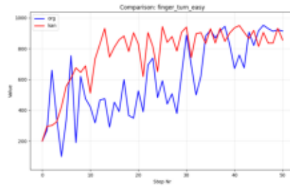
Comparison_finger_turn_easy.png
