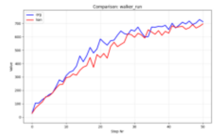
Comparison_walker_run.png
