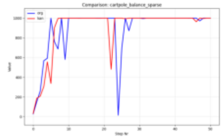
Comparison_cartpole_balance_sparse.png
