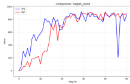
Comparison_hopper_stand.png
