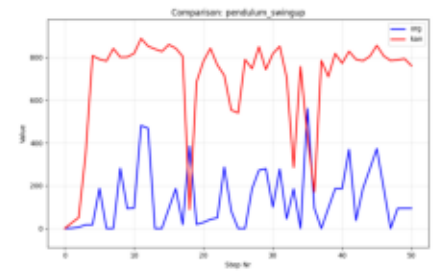
Comparison_pendulum_swingup.png
