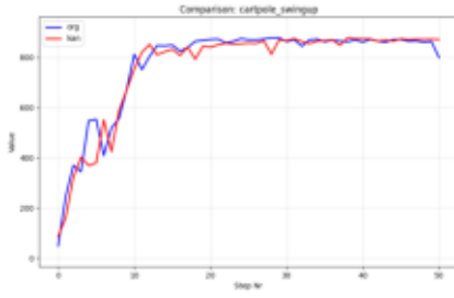
Comparison_cartpole_swingup.png
