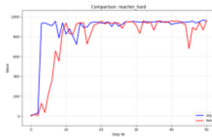
Comparison_reacher_hard.png
