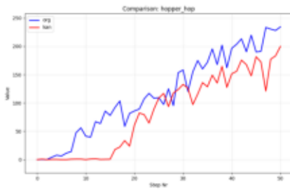
Comparison_hopper_hop.png
