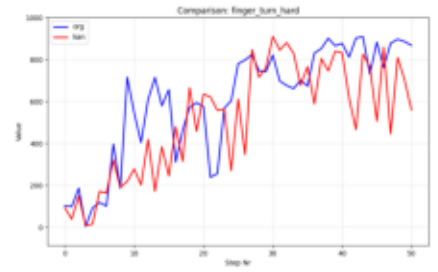
Comparison_finger_turn_hard.png
