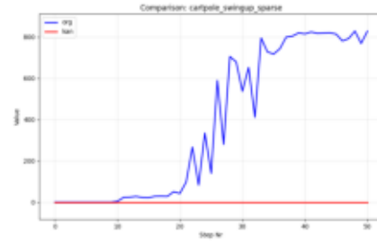
Comparison_cartpole_swingup_sparse.png
