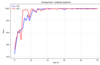
Comparison_cartpole_balance.png
