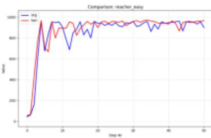
Comparison_reacher_easy.png
