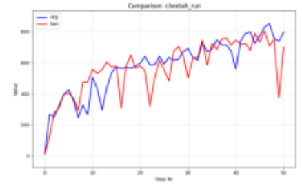
Comparison_cheetah_run.png
