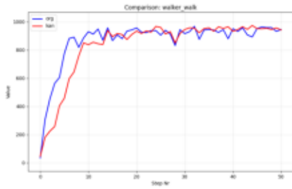
Comparison_walker_walk.png
