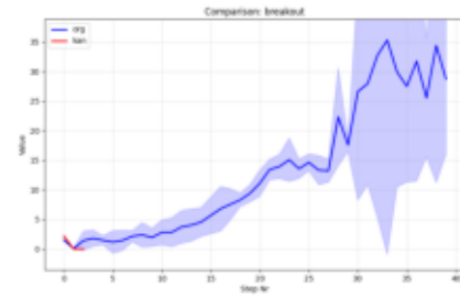
Comparison_breakout.png
