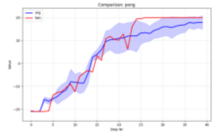
Comparison_pong.png
