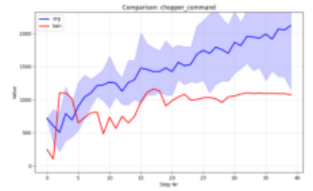
Comparison_chopper_command.png
