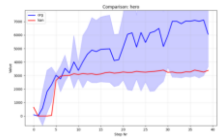
Comparison_hero.png
