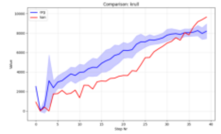
Comparison_krull.png
