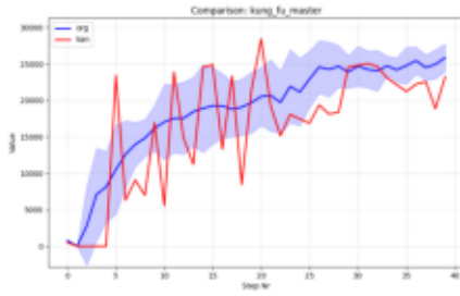
Comparison_kung_fu_master.png
