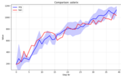
Comparison_asterix.png
