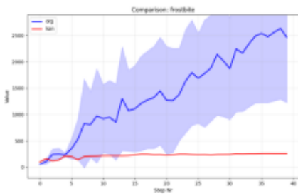
Comparison_frostbite.png
