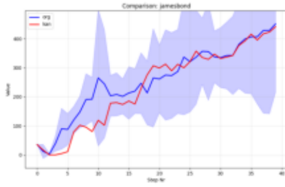
Comparison_jamesbond.png
