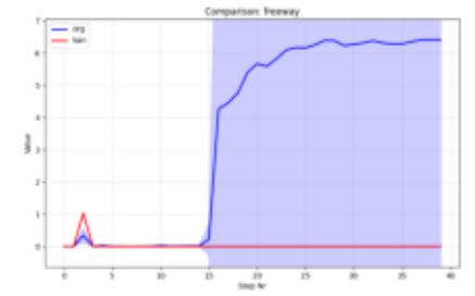
Comparison_freeway.png
