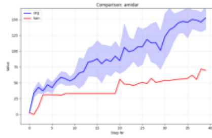
Comparison_amidar.png
