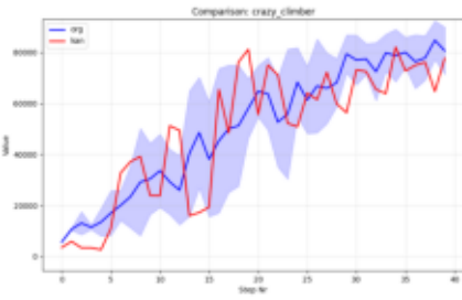
Comparison_crazy_climber.png
