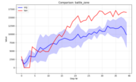
Comparison_battle_zone.png
