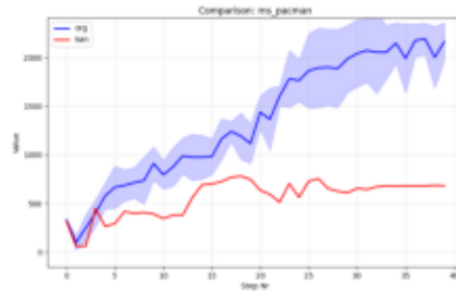
Comparison_ms_pacman.png
