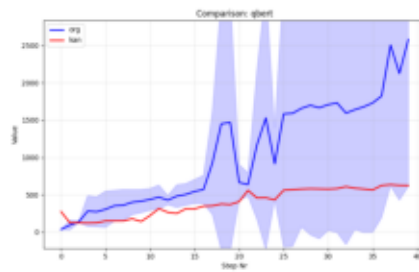
Comparison_qbert.png
