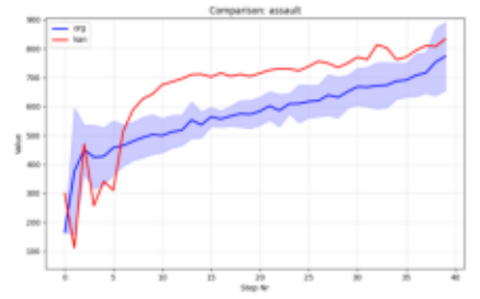
Comparison_assault.png
