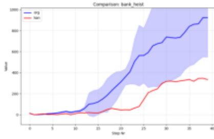
Comparison_bank_heist.png
