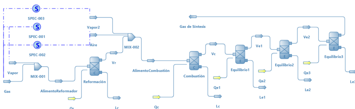
Figura 14.1. Diagrama de flujo de una planta de producción de gas de síntesis.
