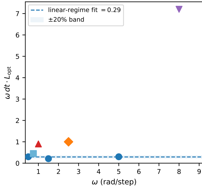
\omega dt \cdot L_{\text{opt}}(\omega)
