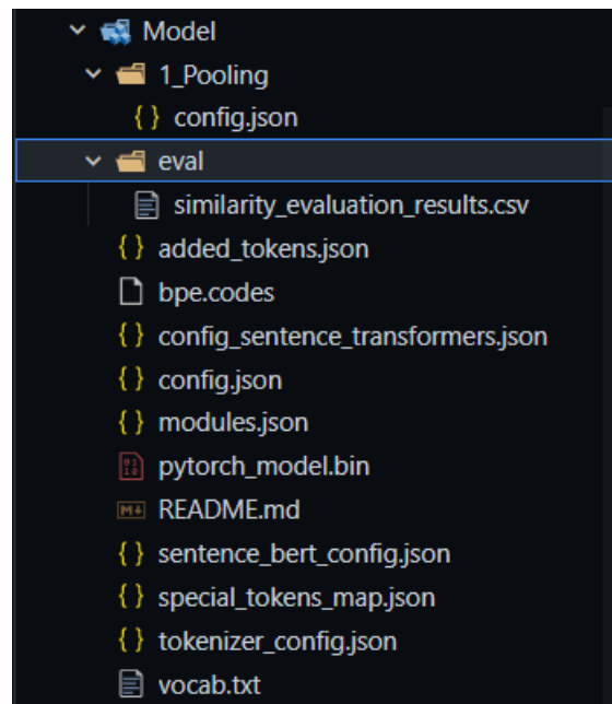
Hình 5.10: Bên trong model mới được trained trên dữ liệu Pháp luật
