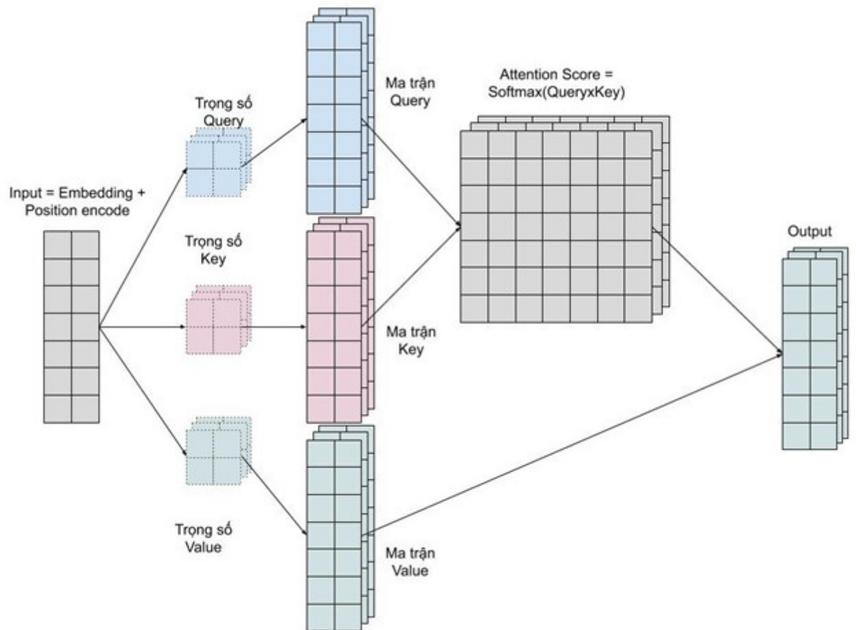
Hình 5.5: Ma trận mã hoá dữ liệu của BERT[10]
