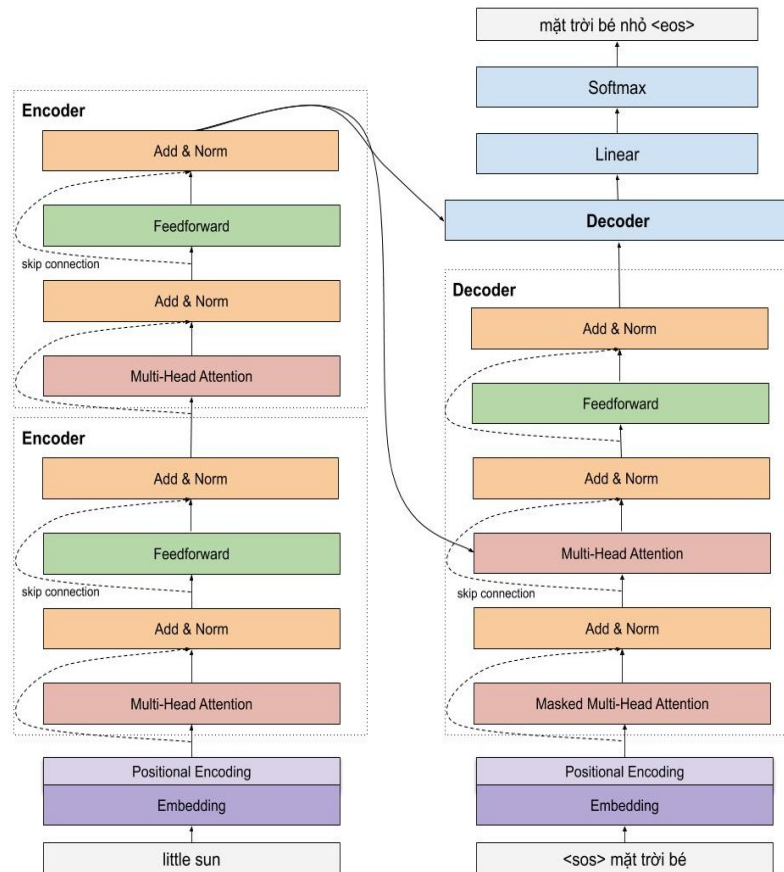
Hình 3.2: Mô hình tổng quát của cấu trúc của Transformer
