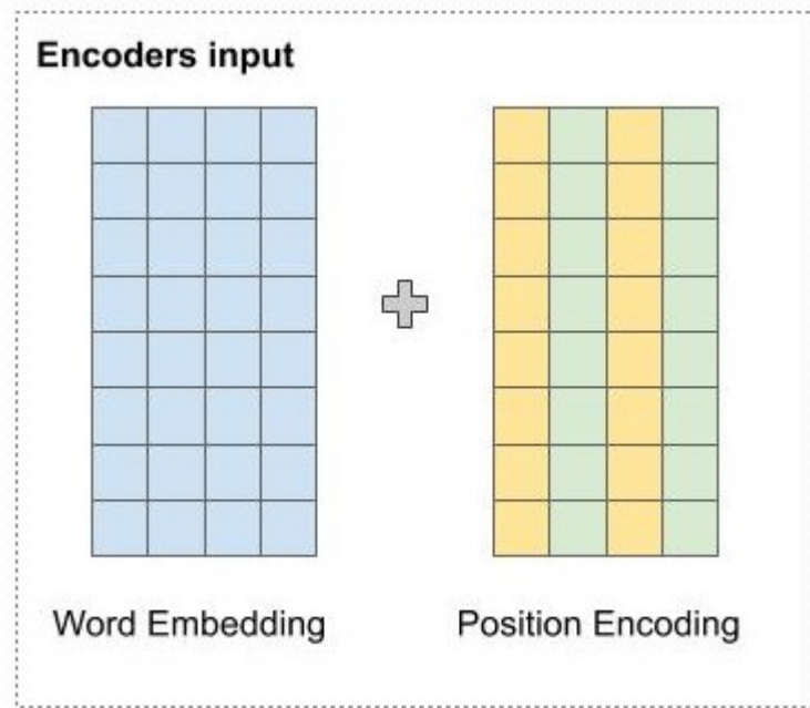
Hình 5.4: Encoders Input
