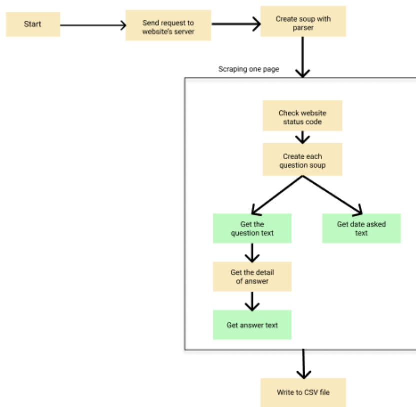
Hình 4.4: Sơ đồ hoạt động của Scraping data từ website
