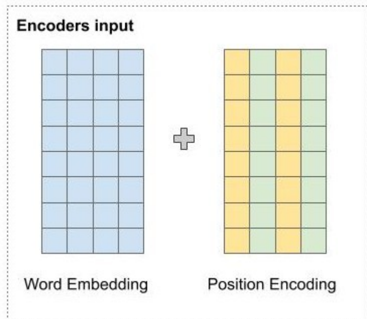
Hình 4.11: Encoders Input
