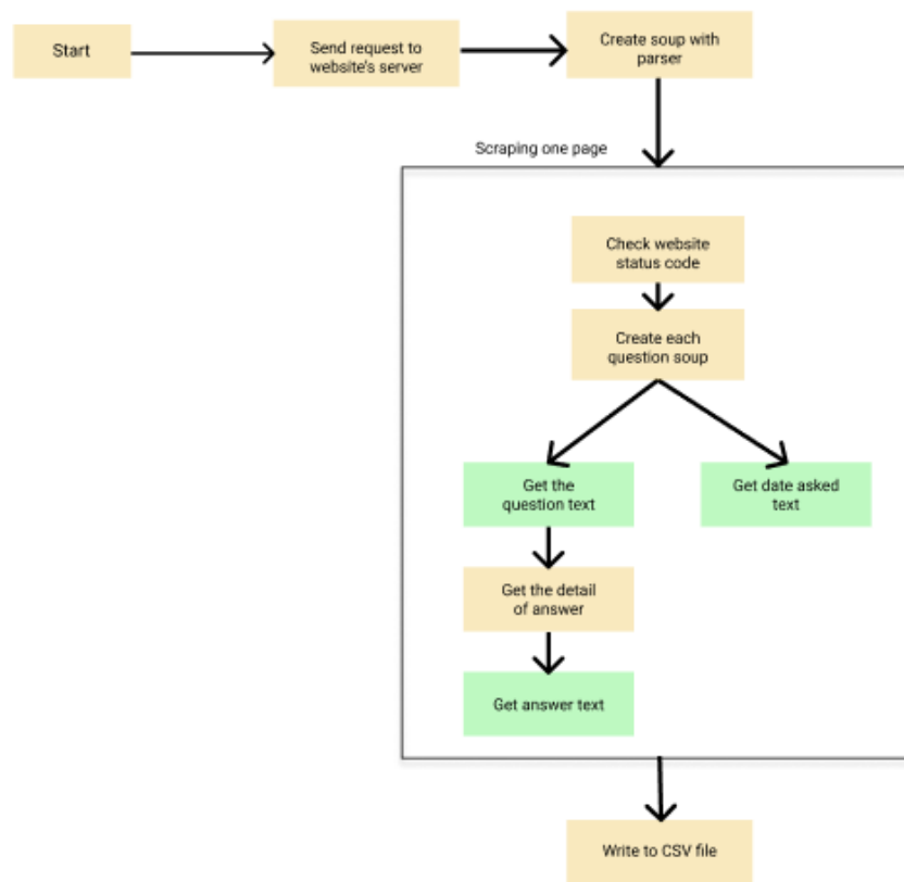
Hình 4.1: Sơ đồ hoạt động của Scraping data từ website
