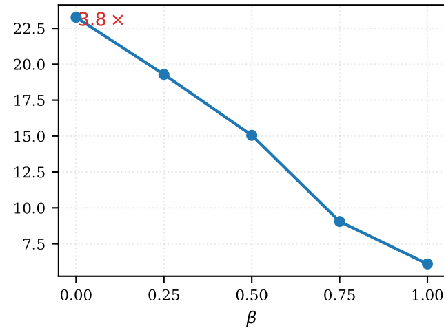
two_moons
