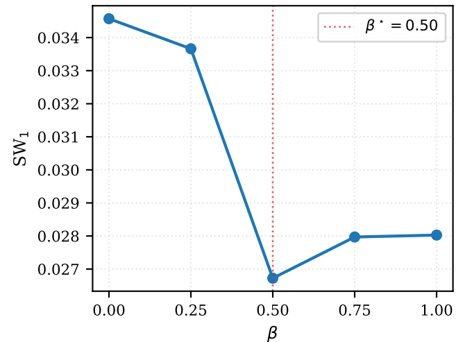
DGMM, d = 64
