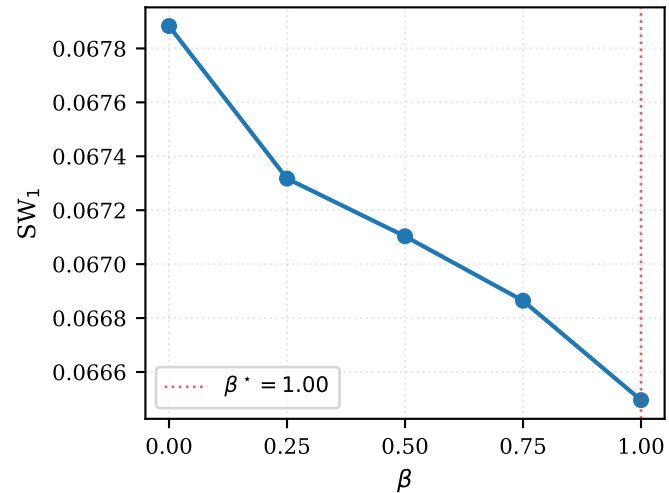
DGMM, d = 8
