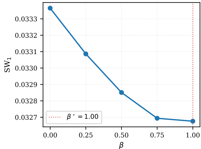
DGMM, d = 32
