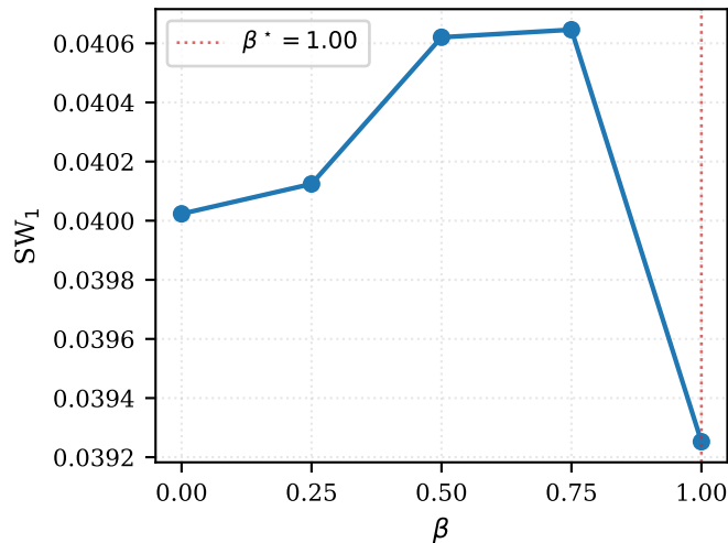
DGMM, d = 16
