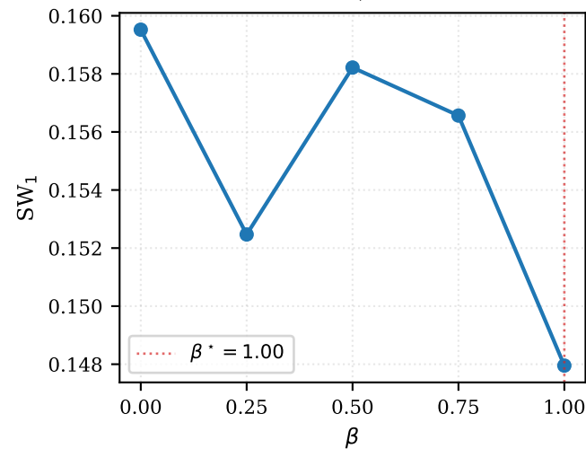
DGMM, d = 2
