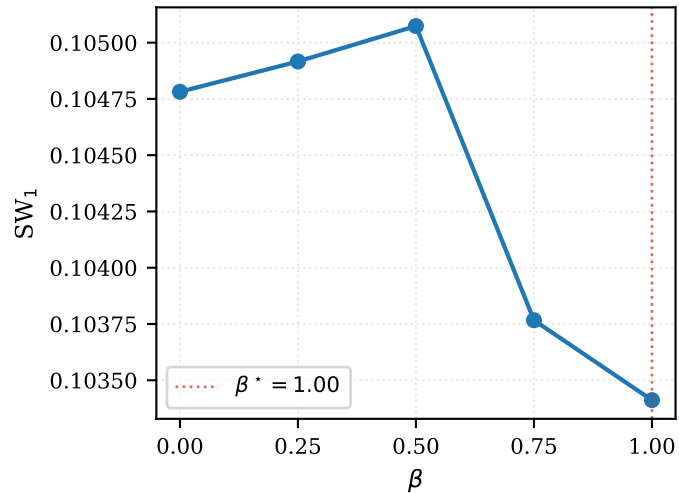
DGMM, d = 4
