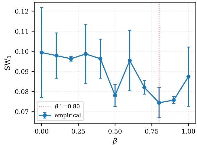
two_moons
