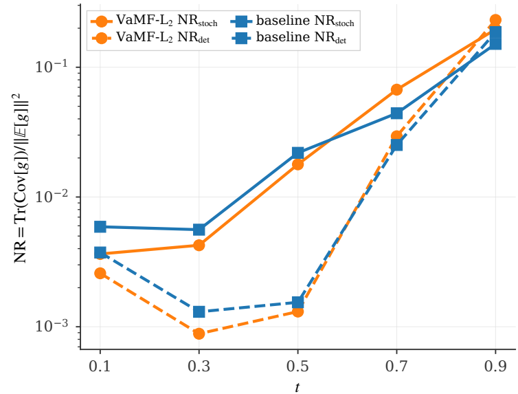
(c) Gradient NR vs t (step 40k)
