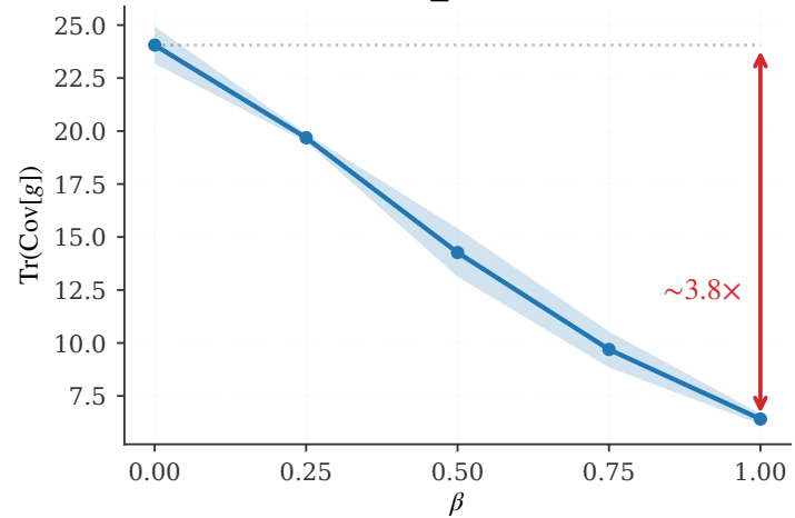
two_moons
