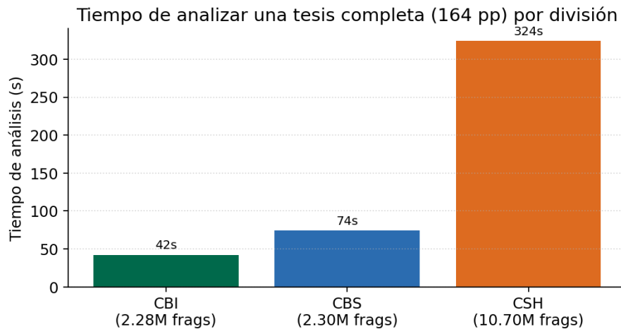
Figura 6.5: Tiempo de análisis por división. El costo crece con el tamaño del corpus (CSH, 10.7M de fragmentos), dominado por la capa de recuperación léxica y de carga única.
