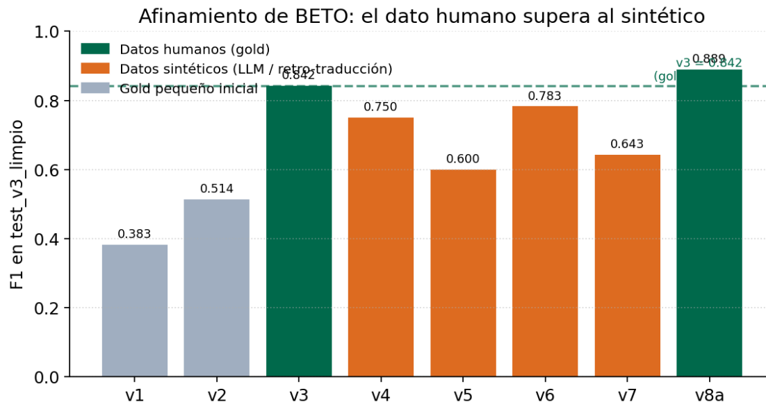
Figura 6.3: Progresión del afinamiento de BETO. Las versiones con datos humanos (v3, v8a, verde) superan a las sintéticas (v4–v7, naranja); ninguna ampliación sintética rebasa la línea del gold humano de v3.
