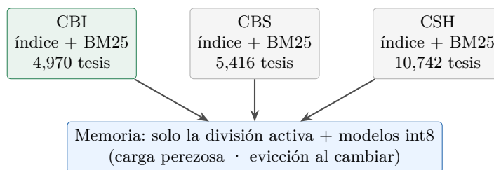
Figura 5.4: Sistema por divisiones. Cada división tiene sus propios artefactos; solo la activa reside en memoria, cargándose de forma perezosa y liberándose al cambiar.
