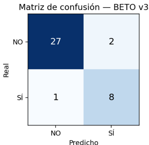
Figura 6.2: Matriz de confusión de BETO v3 sobre test_v3_limpio (38 pares). De 9 positivos reales detecta 8 (un falso negativo) y comete 2 falsos positivos: precisión 0.80, recall 0.889 y F1 = 0.842 .
