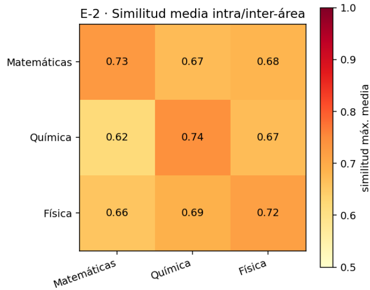
Figura 6.4: Similitud media intra- e inter-área (experimento E-2). La diagonal (misma área) es mayor que fuera de ella, pero el solapamiento entre áreas distintas es considerable ( \sim 0.62 – 0.69 ): confirma que la similitud es afinidad temática, y justifica que un modelo por dominio no aporte.
