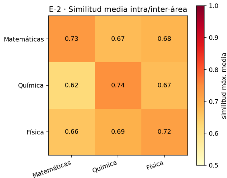
Figura 6.7: Similitud media intra- e inter-área (experimento E-2). La diagonal (misma área) es mayor que fuera de ella, pero el solapamiento entre áreas distintas es considerable (~0.62–0.69): confirma que la similitud es afinidad temática, y justifica que un modelo por dominio no aporte.
