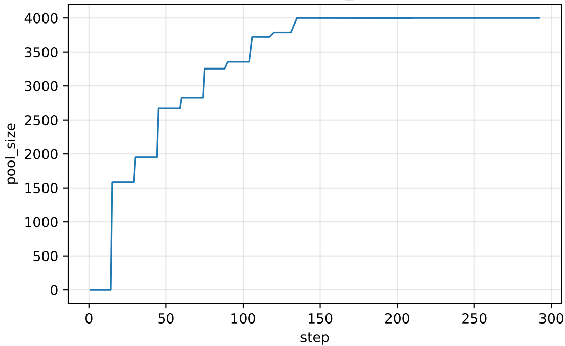
archive/pool_size
