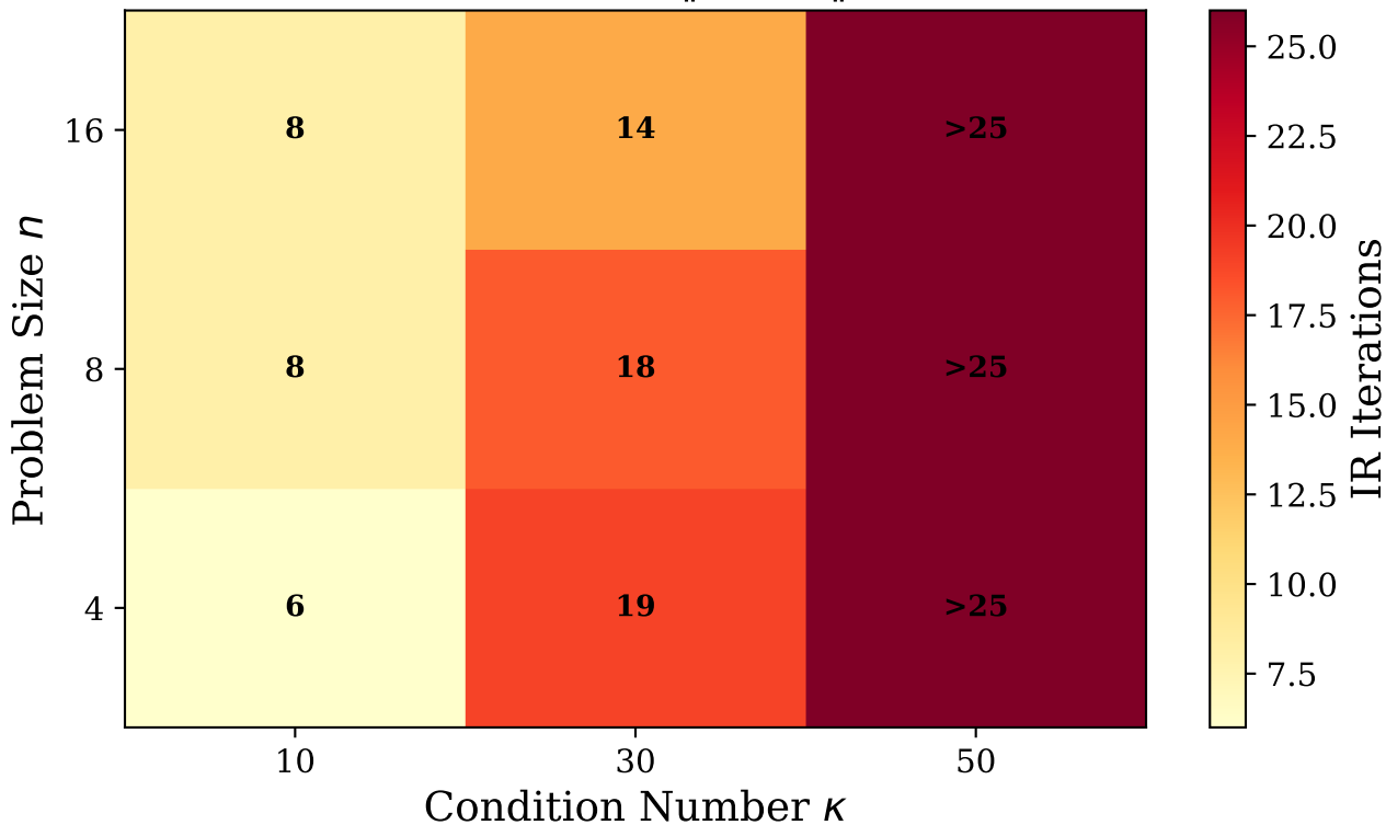
Median IR Iterations to \|Ax - b\|_2 \leq 1e - 05
