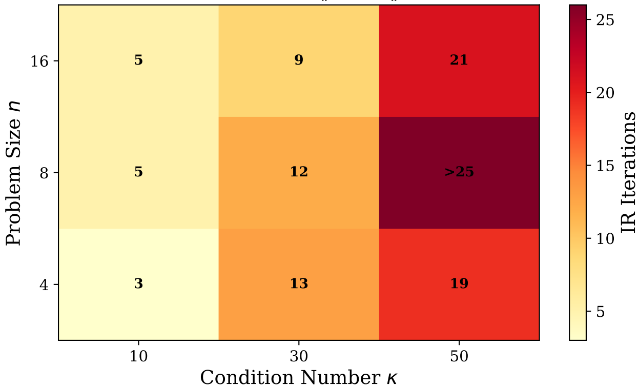
Median IR Iterations to \|Ax - b\|_2 \leq 1e-03
