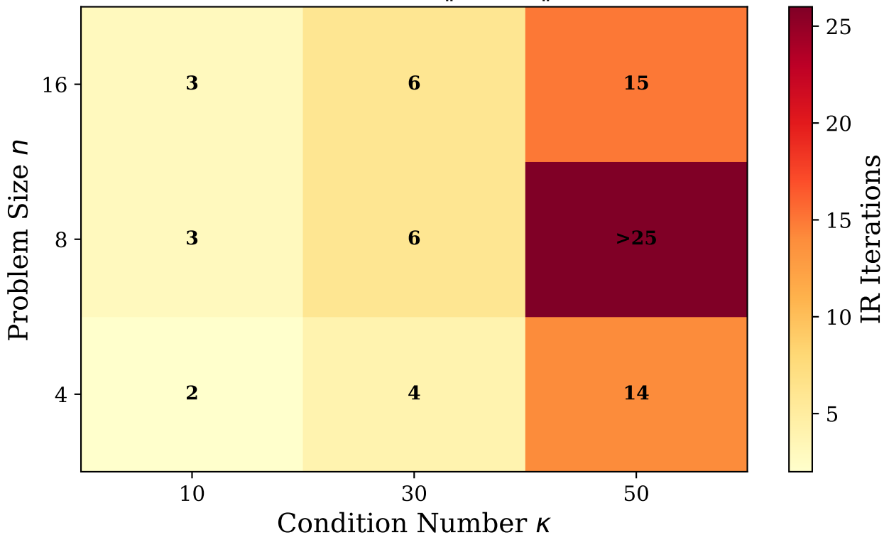
Median IR Iterations to \|Ax - b\|_2 \leq 1e-02
