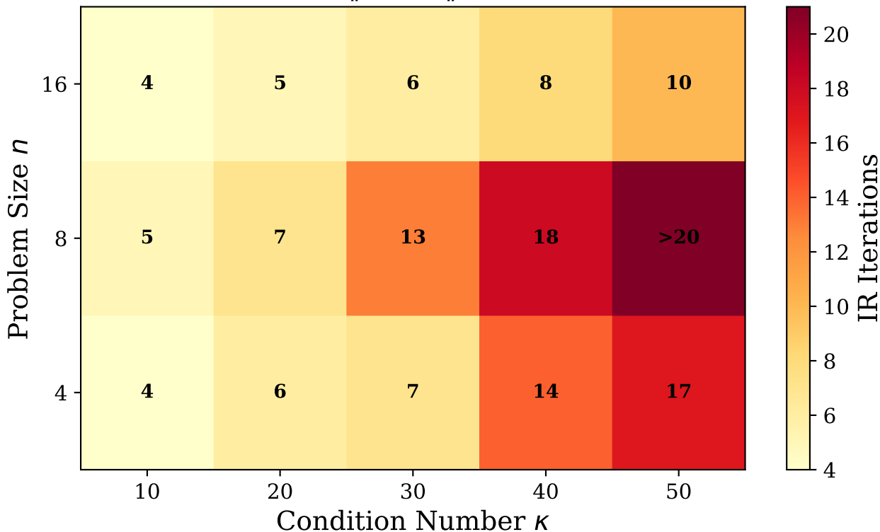
Median IR Iterations to \|Ax - b\|_2 \leq 1e-03 (over 5 seeds)
