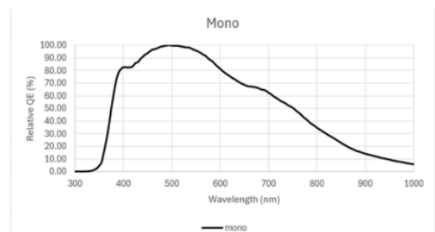
MV-CS050-80UM
