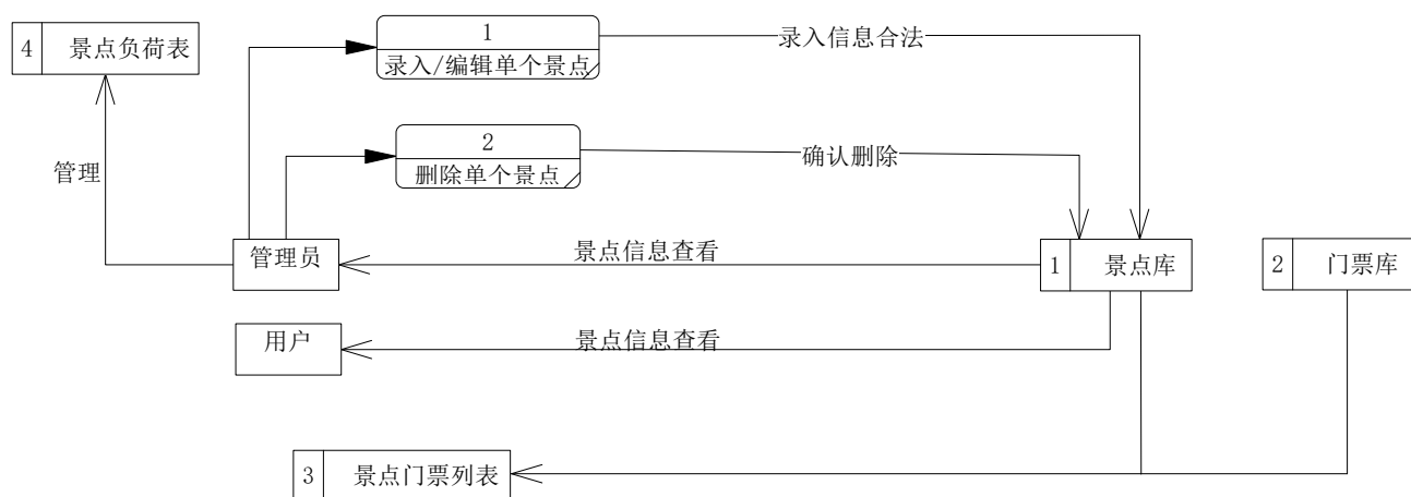
2th DFD 景点信息管理
