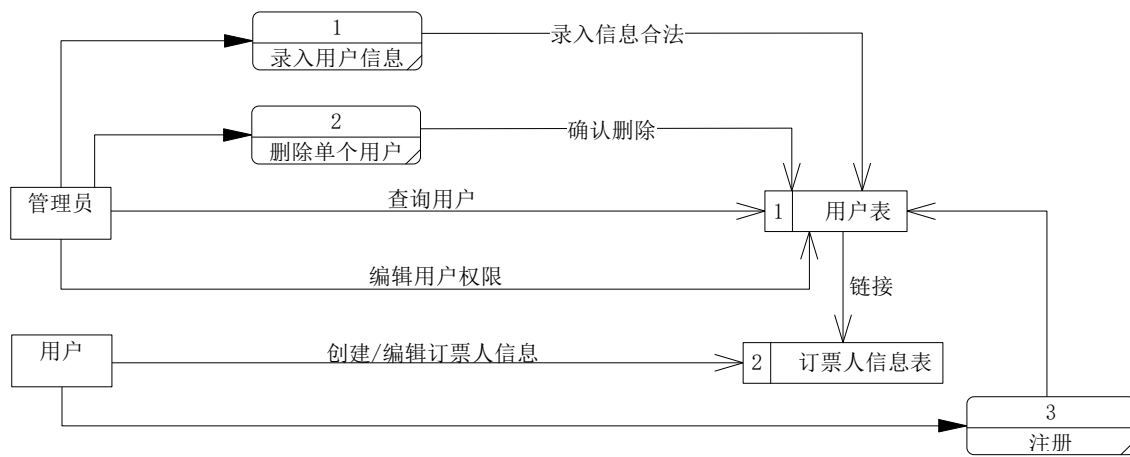
2th DFD 用户信息管理
