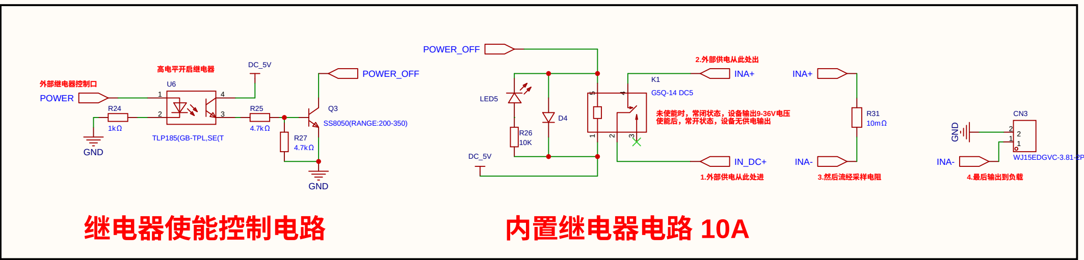
INA226_继电器供电监测
