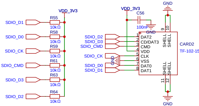
TF-SD存储卡座
