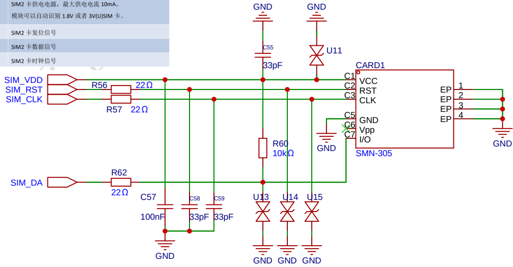
SIM卡
