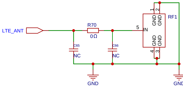
4G LTE天线接口
