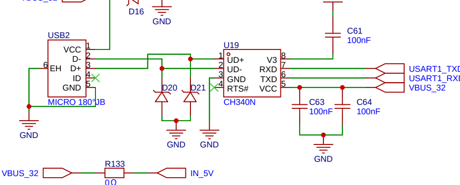
数据观察口USB-CH340（串口1）
