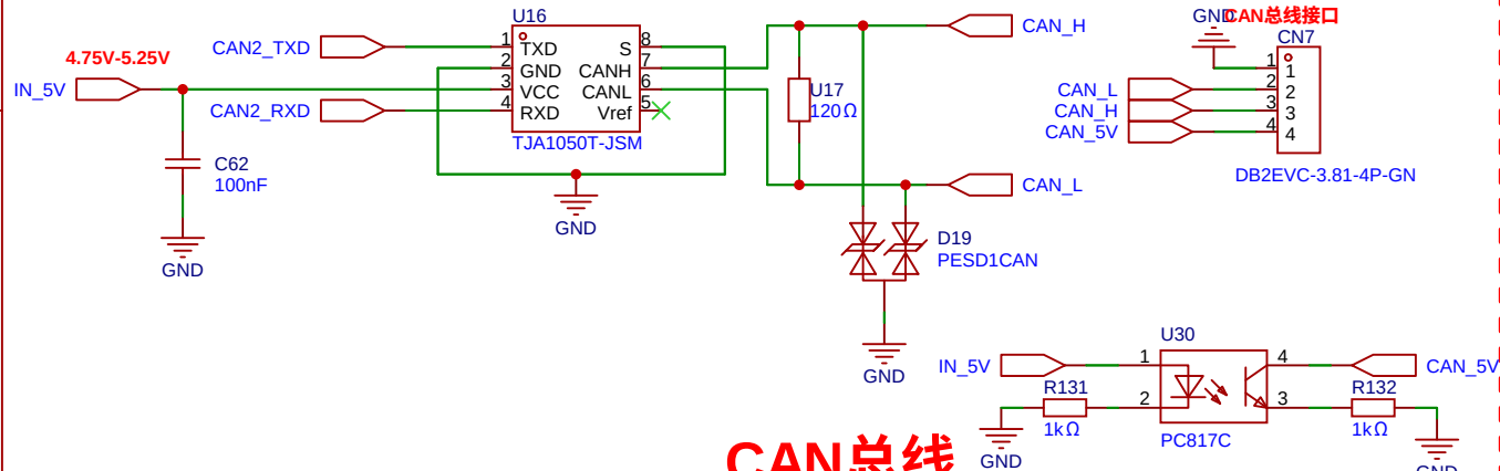
CAN总线
