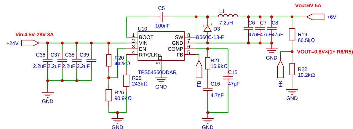
DC-DC 24V to 6V 5A 电机供电电路
