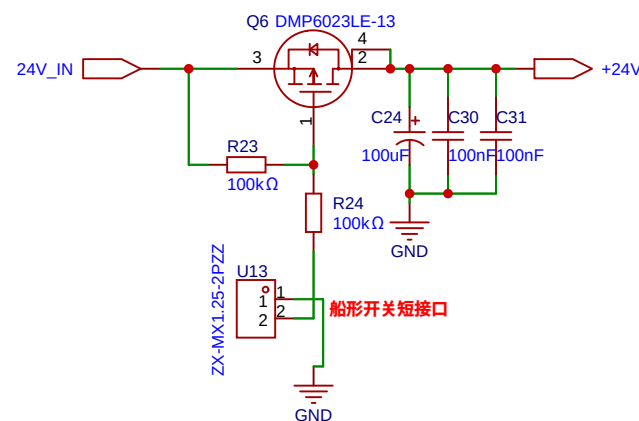
船型开关启动
