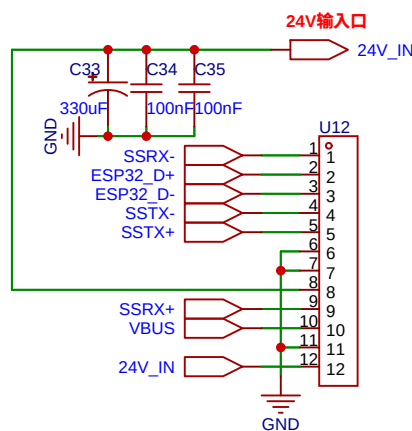
M12航空插 12芯
