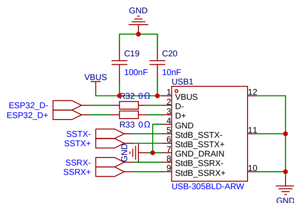
USB3.0接口
