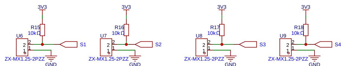
限位触发电路
