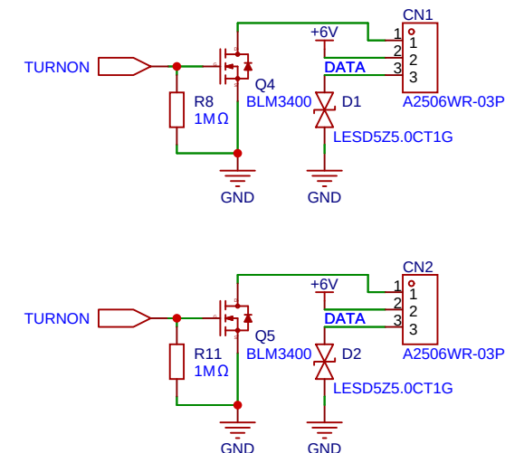
电机使能&接口电路
