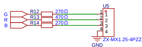
RBG设备状态灯
