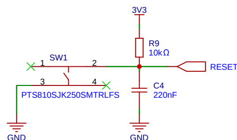
复位电路
