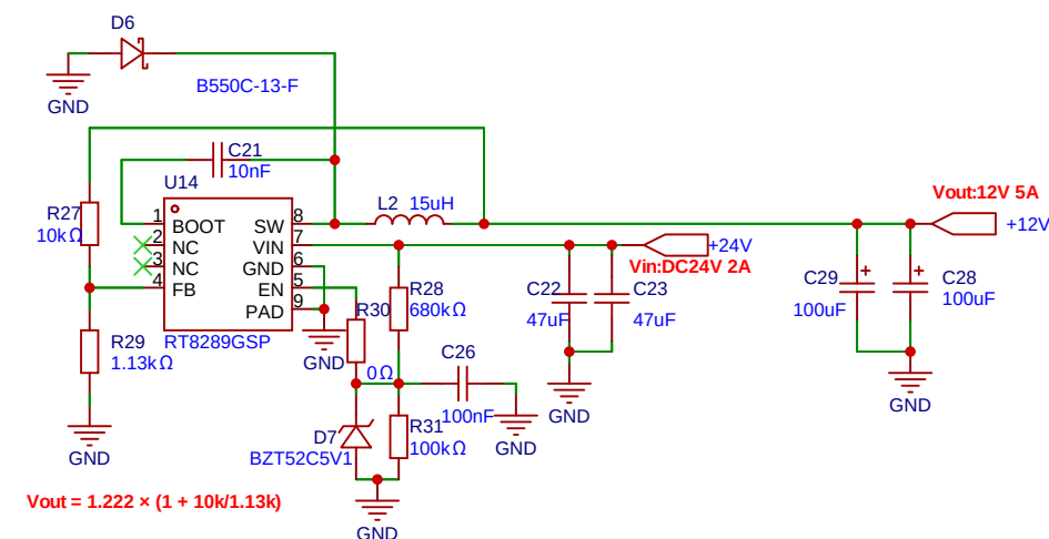
DC-DC 24V to 12V 5A 相机机供电电路
