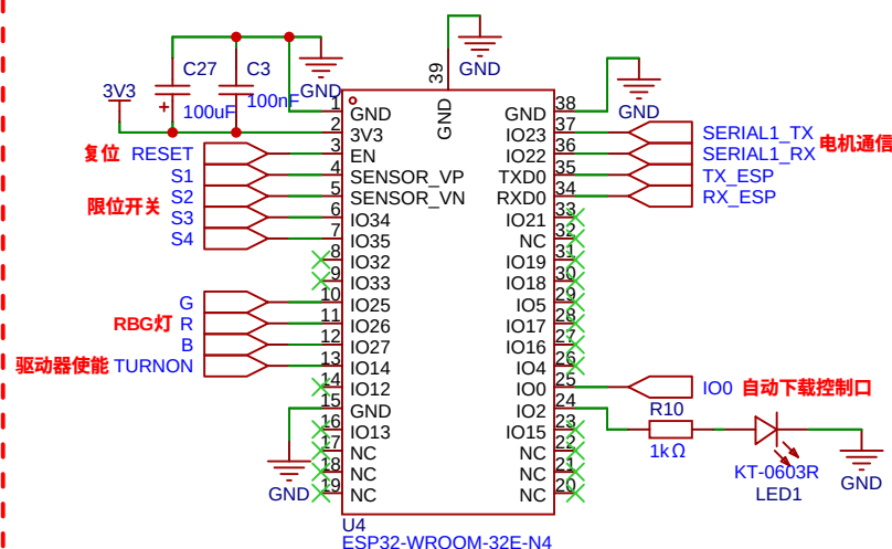
ESP32-WROOM-32E-N4
