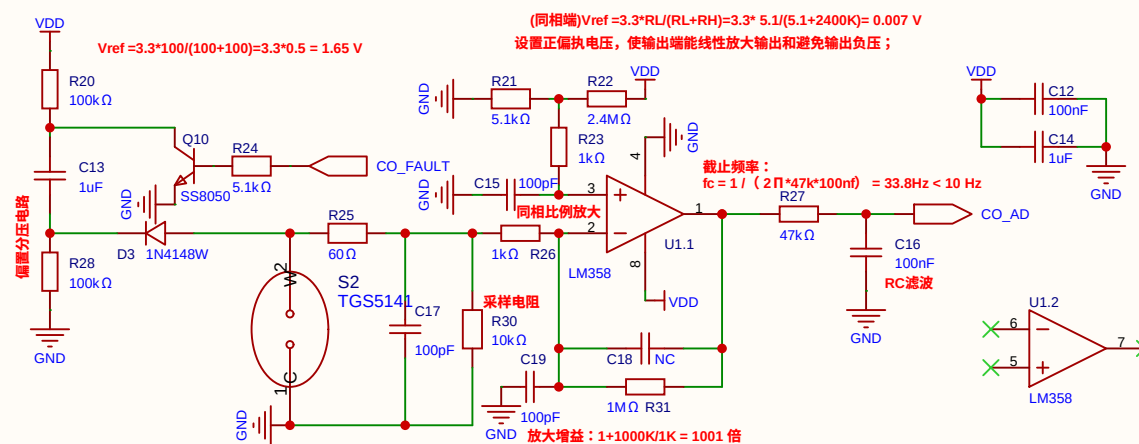
一氧化碳CO 检测采样放大电路
