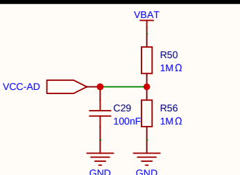
电源状态检测
