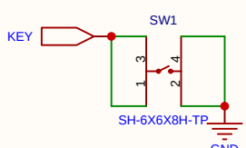
用户按键
