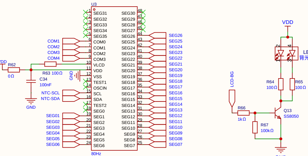
LCD 驱动电路
