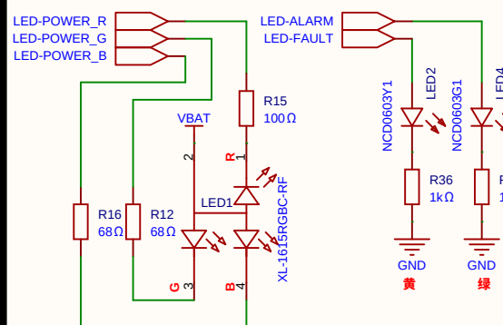
状态显示灯
