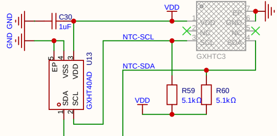
温湿度传感器
