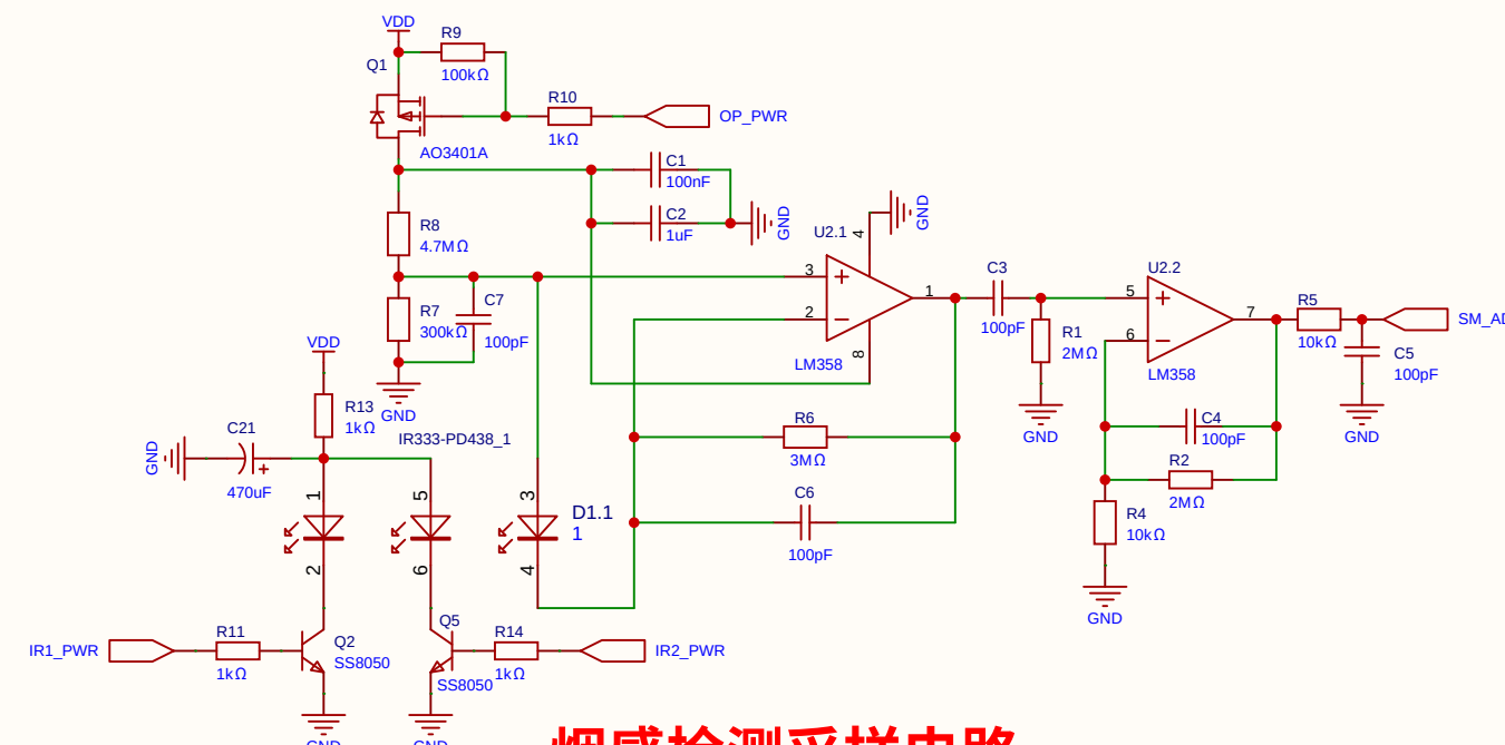
烟感检测采样电路
