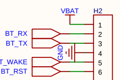
BLE短接口
