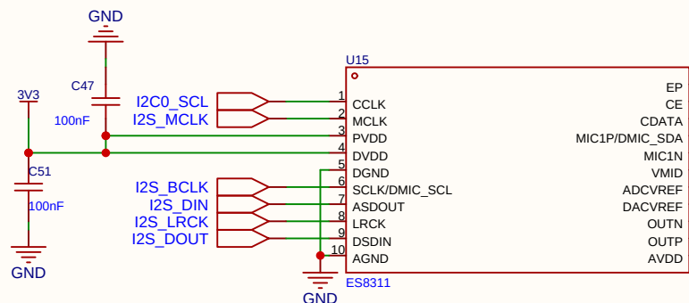
8311_音频芯片 (TTS、MP3)
