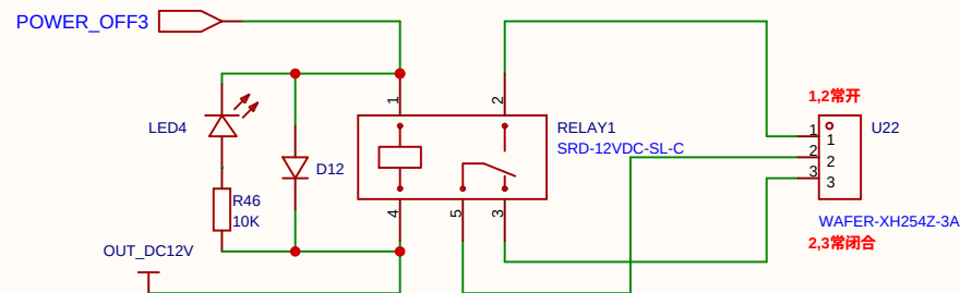
内置12V继电器
