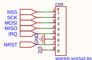
备用RFID读写模块接口-SPI
