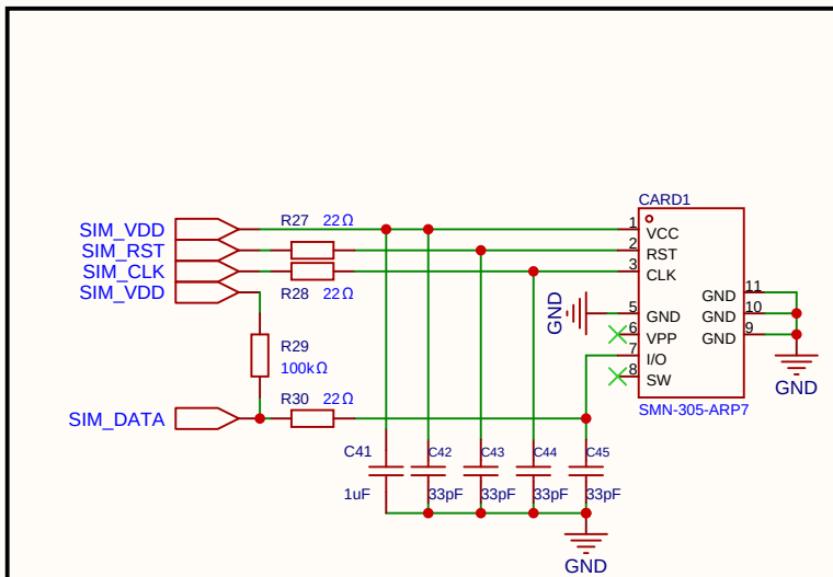
SIM
