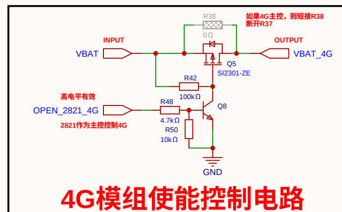
4G-BOOT
