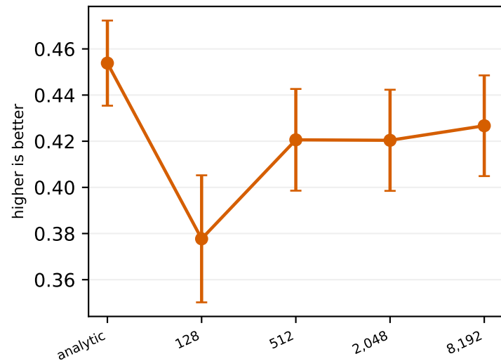
Macro-F1
