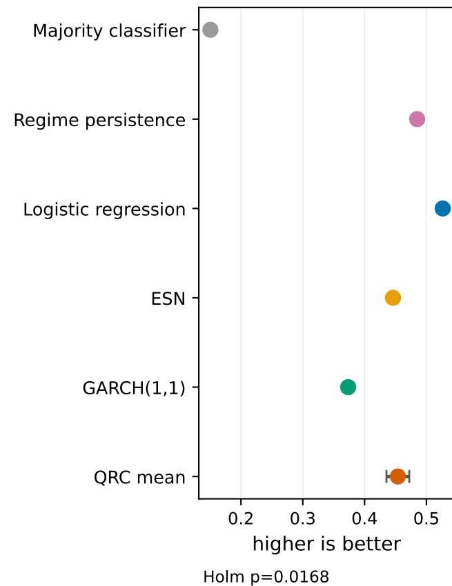
Macro-F1
